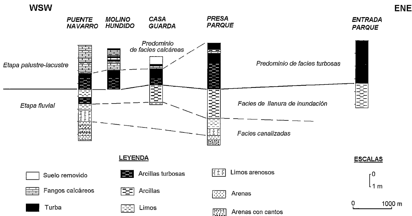
Fig. 2.- Diagrama de correlación litológica y distribución de facies.
