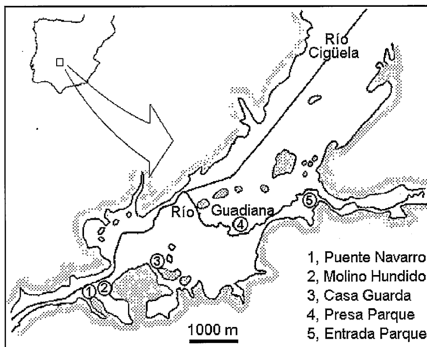
Fig. 1.- Localización geográfica del área estudiada y posición de los sondeos.
