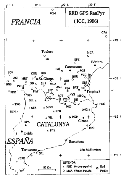
Fig. 1.- Diseño de la red de control geodinámico del Pirineo.
