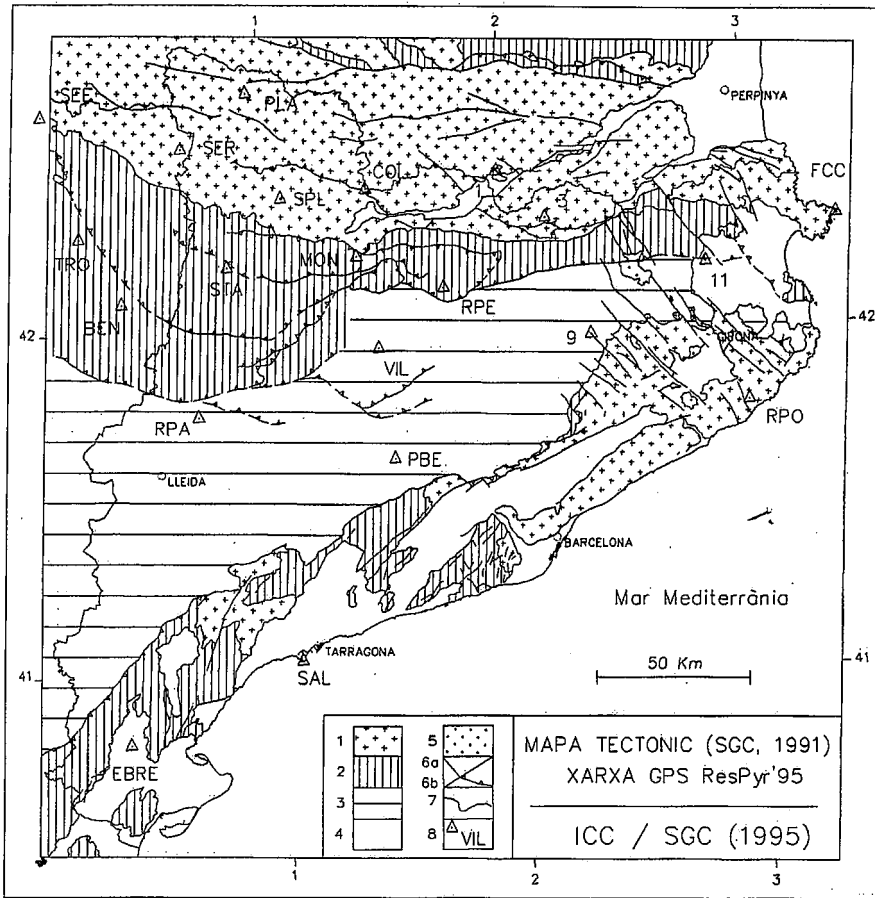
Fig. 2.- Red GPS ResPyr'95 dentro del contexto geológico y estructural de Catalunya. Leyenda: 1. Paleozoico, 2. Unidades alóctonas de cobertera, 3. Cuenca de antepaís, 4. Fosas neógenas, 5. Volcanismo Neógeno y Cuaternario, 6a. Falla, 6b. Cabalgamiento, 7. Contacto litológico, 8. Señal geodésica y nombre.
