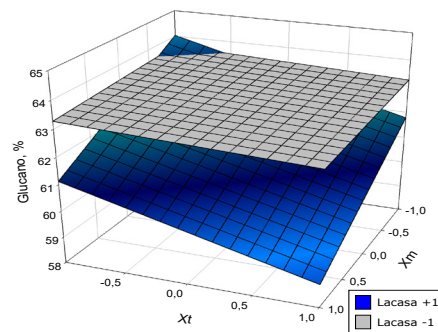
Figura 2: Variación de Glucano según el tiempo de operación y la concentración del mediador (siringaldehído) en dos niveles de concentración de lacasa.
