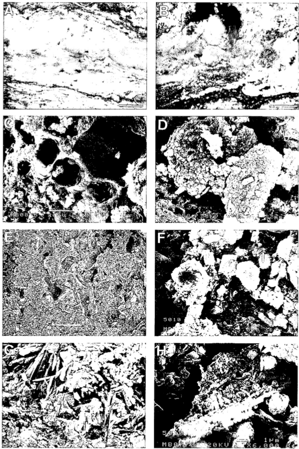
Fig. 2.— A y B: Aspecto de la disposición de los elementos orgánicos fluorescentes, algas interestratificadas con la matriz mineral y colonias de Botryococcus más o menos deformadas (escala= 500 mm). C: Detalle de los poros esféricos relacionados con la liberación de CO 2 y CH 4 durante la fermentación bacteriana (la flecha blanca indica lepisfera de "ópalo-CT" y la flecha negra rombo de ankerita). D: Pellets micríticos de posible origen algal o bacteriano. E: Porosidad móldica originada por la disolución de restos vegetales y conchas en una matriz arcillosa compuesta por interestratificados de Cl-E. F: Rombos ricos en Ca, Mg, Fe, Cr y Cu reemplazando a los pellets calcítico-aragoníticos (el aragonito está marcado por una flecha). G: Fibras y láminas de aragonito reemplazando pellets algales o bacterianos y una morfología globular de Botryococcus . H: Pellet micrítico aragonítico de probable origen bacteriano reemplazandose por rombos de ankerita (flecha).
