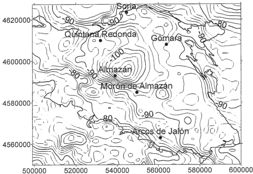
Fig. 2. Mapa de anomalía de Bouguer de la Cuenca de Almazán. Intervalo 2 mGal. Coordenadas como figura 2A.
