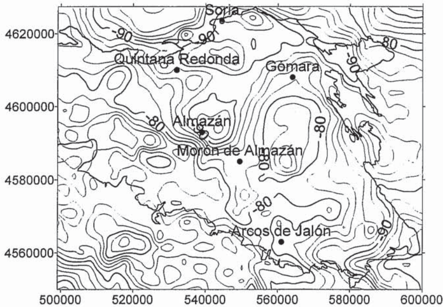
Fig. 4. B) Mapa de anomalía de Bouguer teórica, resultado de restar el efecto que produce la cuenca sedimentaria, con densidad variable en profundidad, al mapa de anomalía de Bouguer. Intervalo 2 mGal. Coordenadas como en figura 2A.
