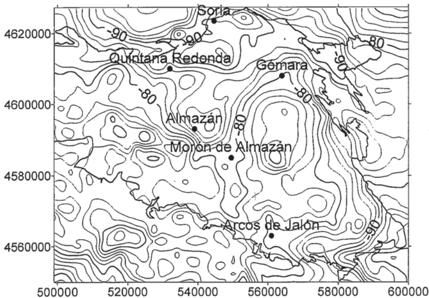
Fig. 4. A) Mapa de anomalía de Bouguer teórica, resultado de restar el efecto que produce la cuenca sedimentaria, con densidad constante en profundidad, al mapa de anomalía de Bouguer. Intervalo 2 mGal. Coordenadas como en figura 2A.
