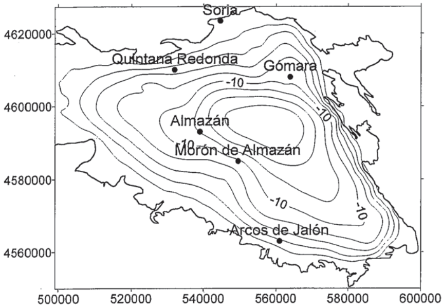
Fig. 3. B) Mapa de anomalía de Bouguer teórica, producida por el relleno sedimentario. Densidad variable de 2.46 gr/cm 3 a 2.69 gr/cm 3 . Intervalo 2 mGal. Coordenadas UTM en metros, huso 30.
