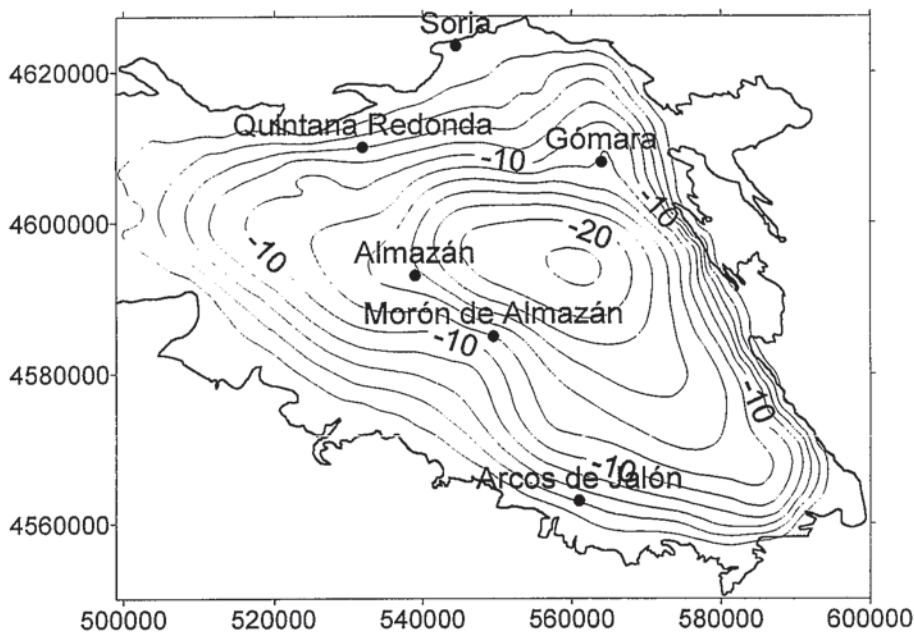
Fig. 3. A) Mapa de anomalía de Bouguer teórica, producida por el relleno sedimentario. Densidad constante 2.51 gr/cm³. Intervalo 2 mGal. Coordenadas UTM en metros, huso 30.
