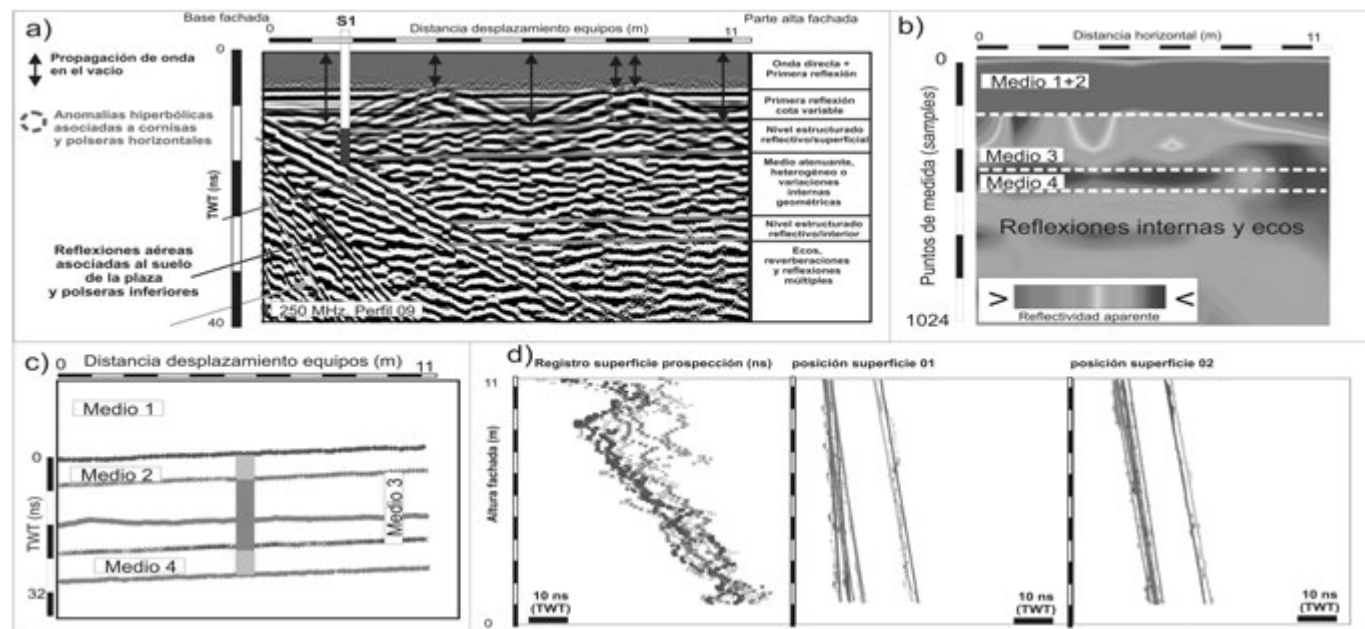
Fig. 2.- a) Perfil de georadar obtenido con el grupo de antenas de frecuencias centrales de 250 MHz con las principales anomalías y unidades geofísicas identificadas. b) Modelo de correlación de reflectividades aparentes para uno de los perfiles obtenidos con el grupo de antenas de 250 MHz (análisis de la reflectividad de los registros). c) Gráfico obtenido del análisis de los registros y de las distintas interfases identificadas en los perfiles (se incluye superpuesto el registro obtenido en uno de los sondeos). d) Representación conjunta de la posición de distintos reflectores o superficies en los distintos perfiles de georadar realizados (previa corrección topográfica). Ver figura en color en la web.
