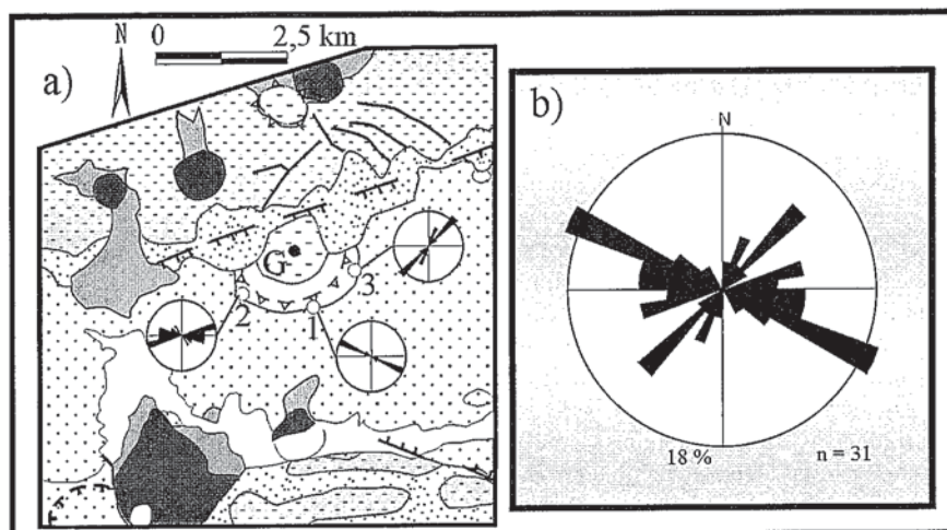
Fig. 2.- a) Situación de los afloramientos estudiados y rosetas de direcciones de las estructuras de licuefacción y b) rosa de direcciones de todas las estructuras estudiadas. Leyenda de la figura 1.
