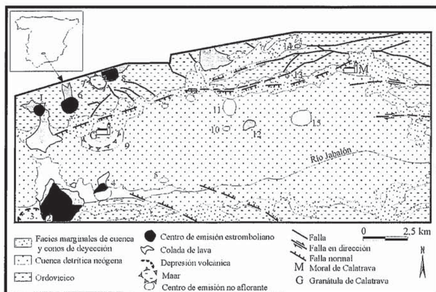
Fig. 1.- Esquema volcano-estructural de la Cuenca de Granátula-Moral. Afloramientos volcánicos: 1. La Cornudilla; 2. La Columba; 3. Casablanca; 4. Las Cuevas; 5. Las Tejas; 6. Cuevas Negras; 7. Maar de la Sima; 8. Cerro Gordo; 9. Maar de Granátula; 10. Tío Ginés; 11. Cantano; 12. Boca del Campo; 13. La Solanilla; 14. Pozo Blanco.
