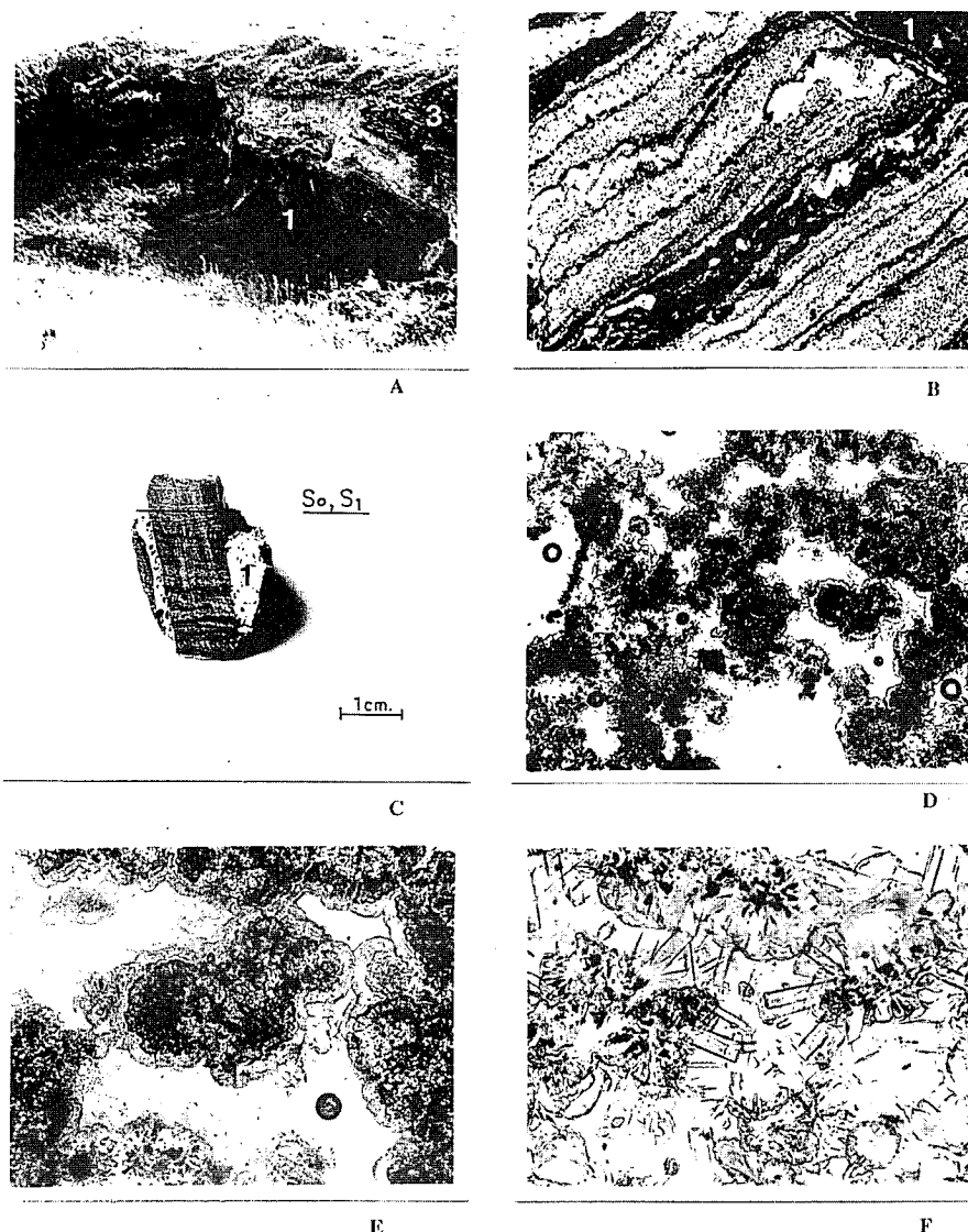
Fig. 2.- (A) Metasedimentos silúricos que afloran en el acantilado de Punta Corveiro (Pontevedra). 1. Liditas, pizarras y cuarcitas negras encajantes de la mineralización. 2. Esquistos moscovíticos muy alterados. 3. Gravas, arenas y arcillas del Pleistoceno. (B) Aspecto microscópico de la textura bandeada y granoblástica milonitizada de las cuarcitas negras encajantes de la mineralización. Obsérvese el estiramiento de los granos de cuarzo y la presencia de un filon-cillo mineralizado (1) (LNx10). (C) Obsérvese la potencia centimétrica de las fracturas mineralizadas (1) y su disposición prácticamente perpendicular a la esquistosidad de la roca. (D) Aspecto microscópico de la textura esferulítica de la mineralización (LNx63). (E) Obsérvese cómo los esferulitos tienen un núcleo de micro a criptocristalino y una periferia lisa, botroidal con un claro crecimiento concéntrico (LNx160). (F) Microfotografía a grandes aumentos (x320) en la que se observa el crecimiento perpendicular de los cristales prismáticos de variscitas en la capa externa de los esferulitos (LNx320).
