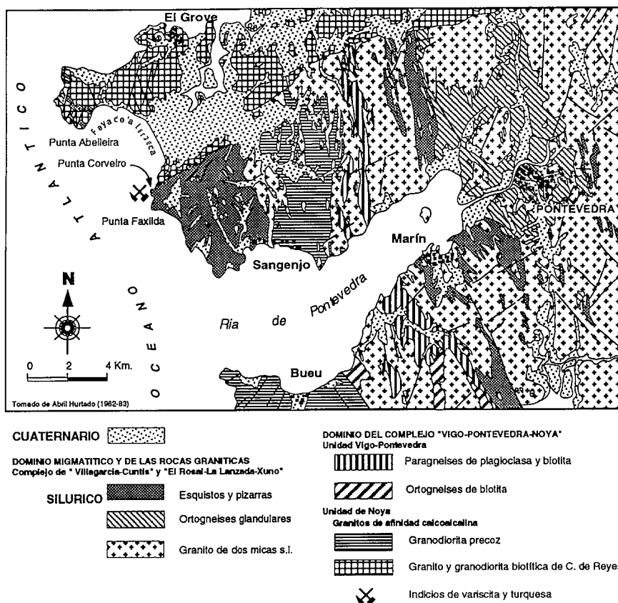
Fig. 1.- Mapa geológico del sector W de la provincia de Pontevedra con la situación del indicio mineralizado (Abril Hurtado, 1982-83).
