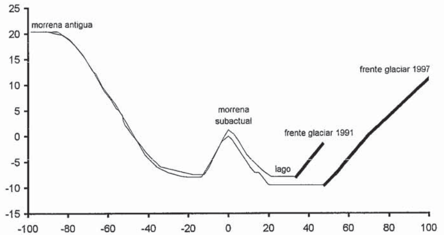
Fig. 3.- Perfiles topográficos del frente del lóbulo BAE, realizados en 1991 y 1997. Ccordenadas locales en metros.
