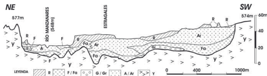
Fig. 2.- Sección morfoestratigráfica del by-pass de la Terraza Compleja de Butarque (TCB) en Peralas del Río, al sur de Madrid. Leyenda: R: vertidos, F/Fa: fango, G/Gr: grava, A/Ar: arena, Y: yeso (Terciario).
