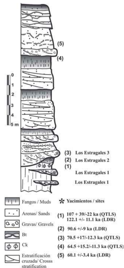
Fig. 3.- Sucesión arqueostratigráfica de Los Estragales en la Terraza Compleja de Butarque (TCB) del valle bajo del río Manzanares, en Perales del Río (Madrid). TL (QTLS: Quaternary TL Surveys, UK) y OSL (LDR: Laboratorio de Datación y Radioquímica, Universidad Autónoma de Madrid).
