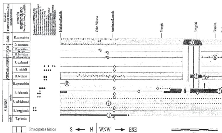
Fig. 3.- Diagrama cronoestratigráfico de los episodios volcánicos y unidades sedimentarias que los engloba. Con rombos se indica la localización de las muestras de campo más representativas del análisis paleontológico desarrollado (basado en foraminíferos planctónicos). En la parte izquierda del diagrama se muestra la distribución vertical de los marcadores bioestratigráficos, lo que justifica su correspondencia con la biozonación de Caron (1985). *1: datación basada en amonites y nanoplankton (texto). *2: datación basada en nanoplankton. *3: datación basada en EVE (1990). Se aplica la misma leyenda de la figura 2.
