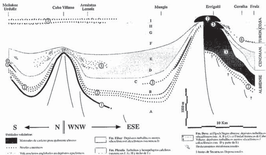
Fig. 2.- Diagrama litoestratigráfico que muestra la distribución espacial de los episodios volcánicos y su relación con paleoaltos submarinos. Secuencias deposicionales: A) S. Jata, B) S. Matxitxako-Armitza, C) S. Larragan, D) S. Cabo Villano, E) S. Lemoiz, F) S. Saratxaga, G) S. Astondo, H) S. Matxilando, e I) S. Arrizabala. Los números representan los sucesivos episodios volcánicos aducidos en el texto. El Episodio Volcánico de Armitza (1) muestra su escala vertical exagerada.
