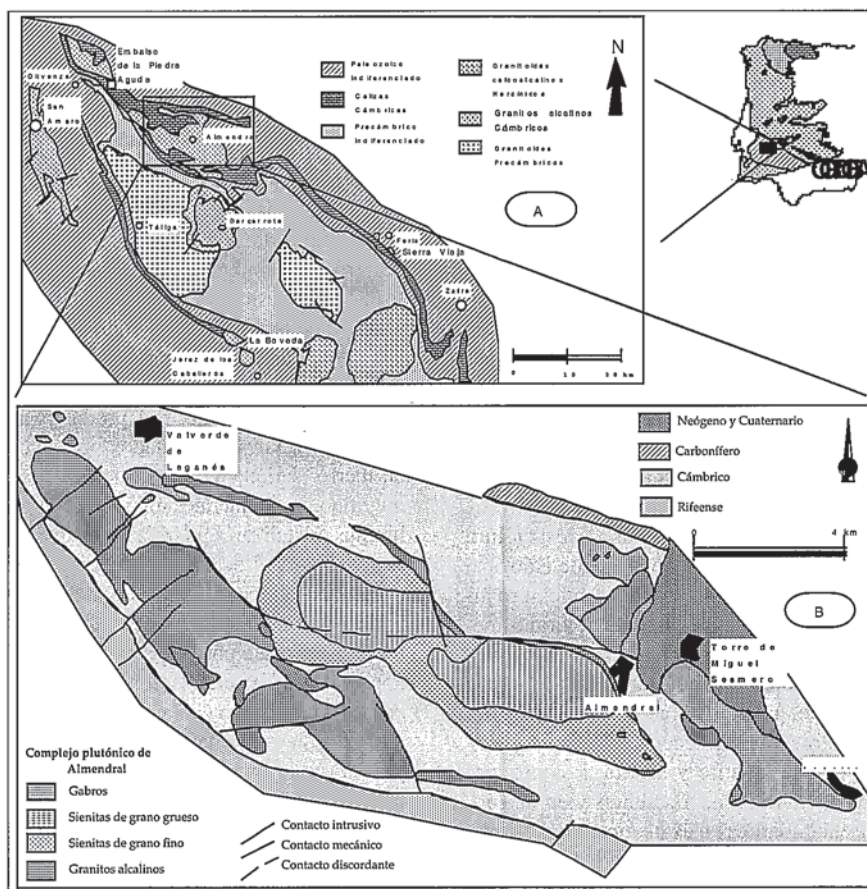
Fig. 1.- Esquema cartográfico que recoge A) la ubicación del Macizo de Almendral en el contexto geológico de la terminación NW de Olivenza-Monesterio (ZOM) y B) la cartografía del Macizo.
