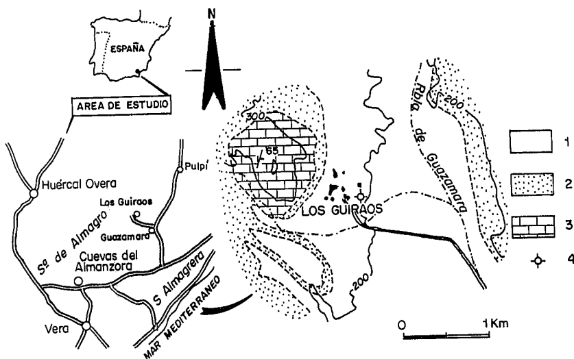
Fig. 1.-Situación geográfica y esquema hidrogeológico del área estudiada. 1: conglomerados, arenas, limos y arcillas (Cuaternario); 2: margas y areniscas (Mioceno); 3: filitas, cuarcitas, calizas, areniscas y diabasas (Pérmico); 4: sondeo. Modificado de Espinosa et al. , 1973.
