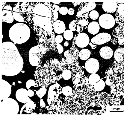
Fig. 2.—Vista en lámina delgada (fotografía en negativo) de las facies en la que se observan los cantos de calizas oolíticas con la matriz con foraminíferos planctónicos.
