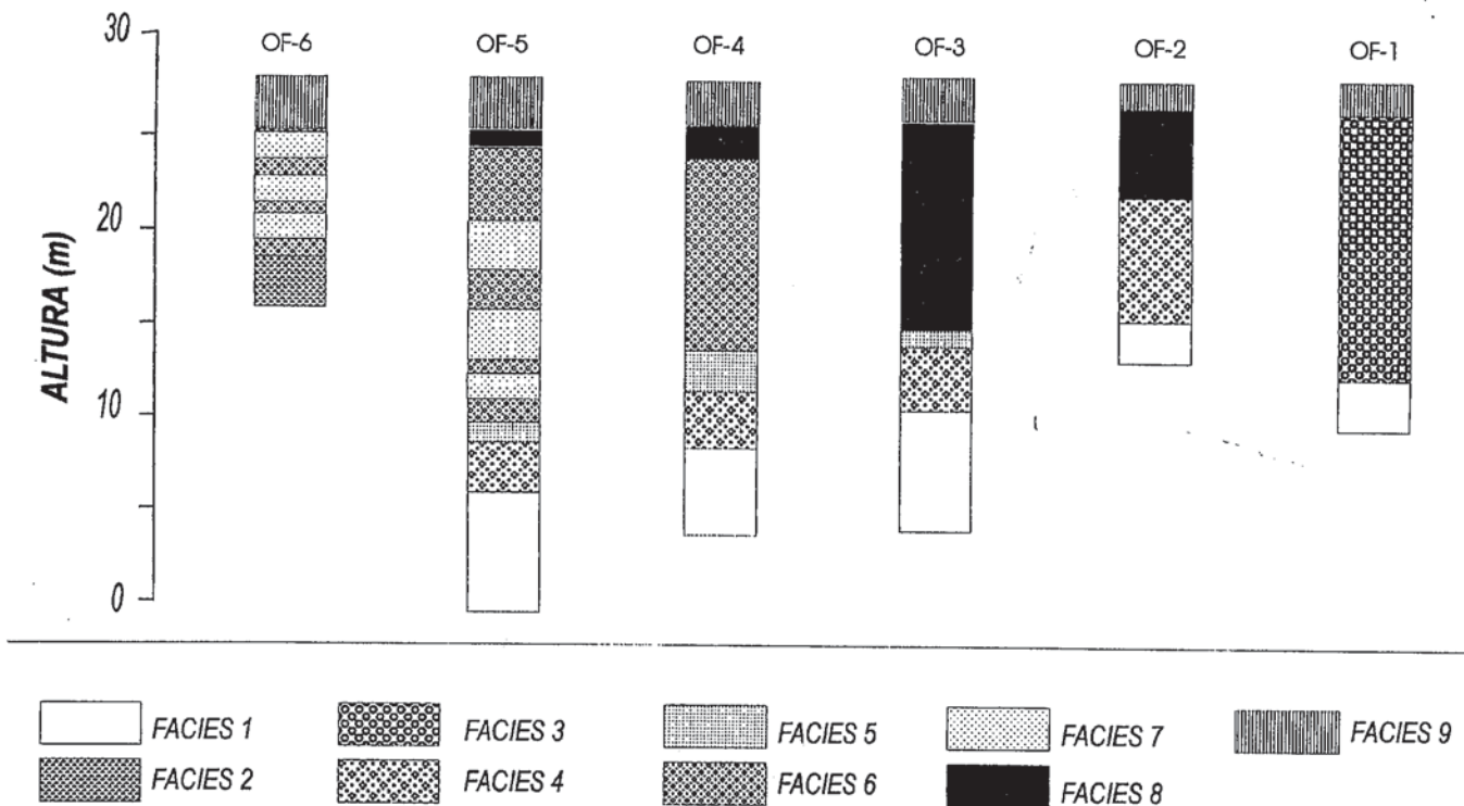
Figura 2.- Secuencia sedimentaria de los seis sondeos estudiados.
