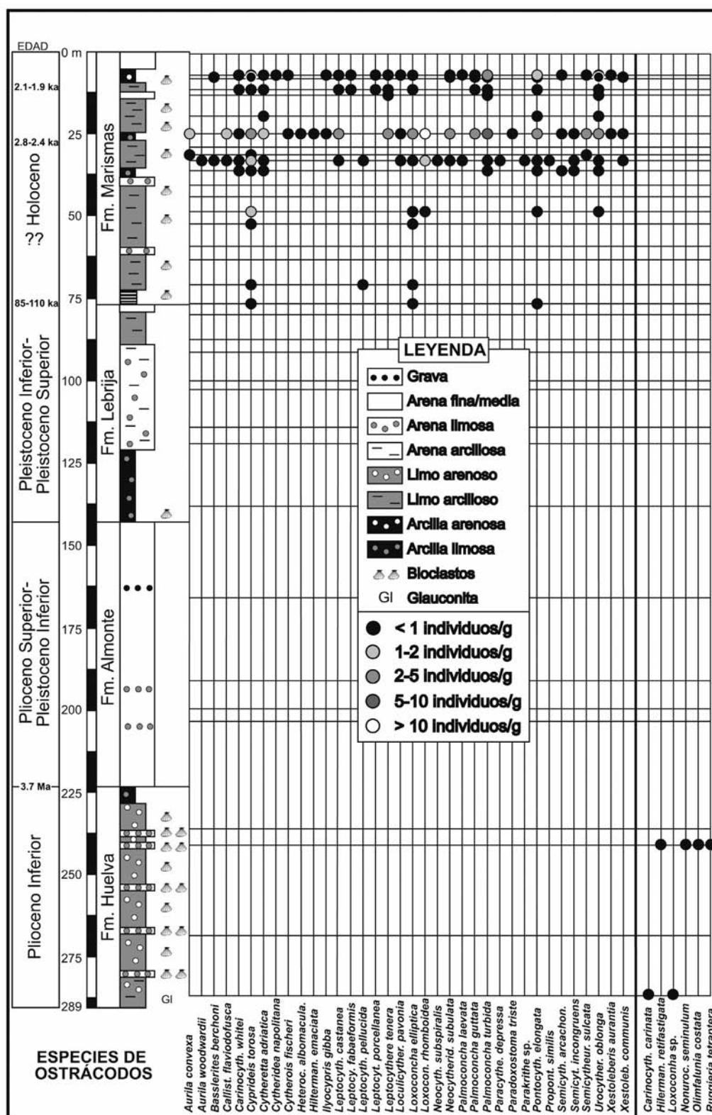
Fig. 2.—Sección sintética del testigo CM (modificada de Salvany et al. (2011) y Rodríguez Vidal et al. (2011), con inclusión de la abundancia relativa de las especies de ostrácodos en las muestras seleccionadas. Edades tomadas de Salvany et al. (2011), excepto las dos superiores (ver metodología). Las líneas horizontales coinciden con las muestras analizadas para el estudio de los ostrácodos.
