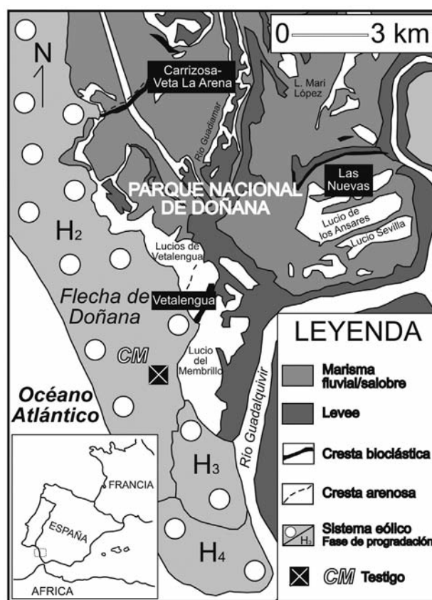
Fig. 1.—Geomorfología general del sector meridional del Parque Nacional de Doñana, con la localización del testigo CM. En negrita, nombre local de determinados sectores del Parque (p.e., Las Nuevas).
