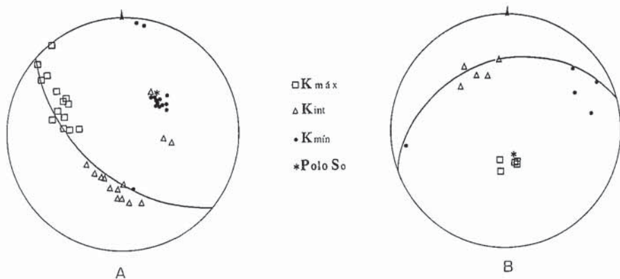
Fig. 2.- Proyecciones estereográficas de los ejes del elipsoide de diversas estaciones de muestreo: (A) Estación 30, los ejes K máx y K int definen prácticamente la traza de S 0 ; mientras que el eje K mín lo hace con el polo de la estratificación. (B) Estación 49, los ejes K int y K mín definen la S 0 , mientras K máx coincide con el polo de la estratificación.
