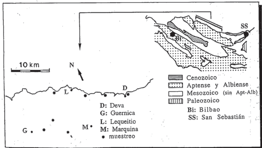
Fig. 1.- Localización de las zonas de muestreo en turbiditas albienses del sector septentrional de la Cuenca Vasco-Cantábrica, entre Guernica (Vizcaya) y Deva (Guipuzcoa).
