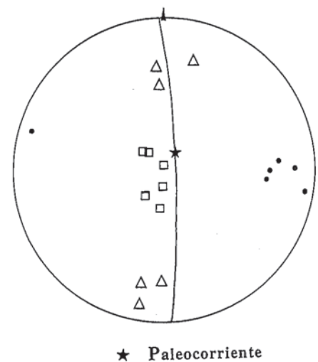
Fig. 5.- Proyección estereográfica de los ejes del elipsoide de las muestras de la Estación 22. Los ejes K_{máx} obtenidos concuerdan mayormente con la dirección de paleocorriente medida directamente en el afloramiento (La simbología no indicada es la misma que la de la Fig. 2).
