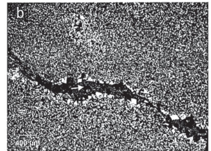
Fig. 3.- Fotomicrografías con nicoles cruzados (las flechas señalan calcita teñida con solución de Rojo de Alizarina): a) Bioesparita dolomitizada b) dolomía microcristalina
