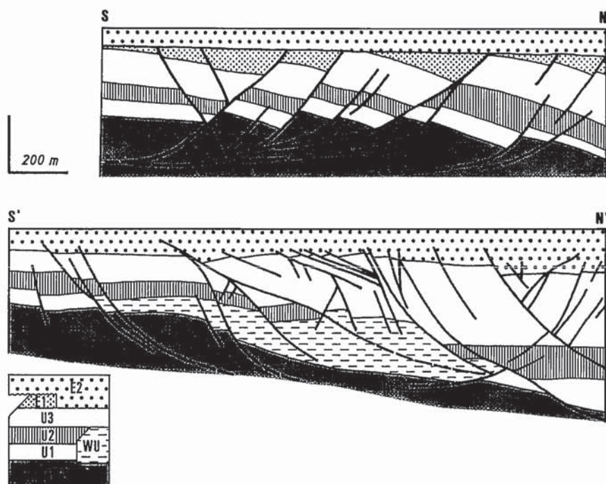
Fig. 4- Cortes interpretativos de la estructura cretácica en ambos flancos del anticlinal de Campos, restituída llevando a la horizontal un nivel de referencia situado en la parte alta de la Fm. Escucha. S-N: flanco oeste; S'-N': flanco este (ver situación en figura 1). Las siglas de la leyenda son las mismas utilizadas en la figura 1.
