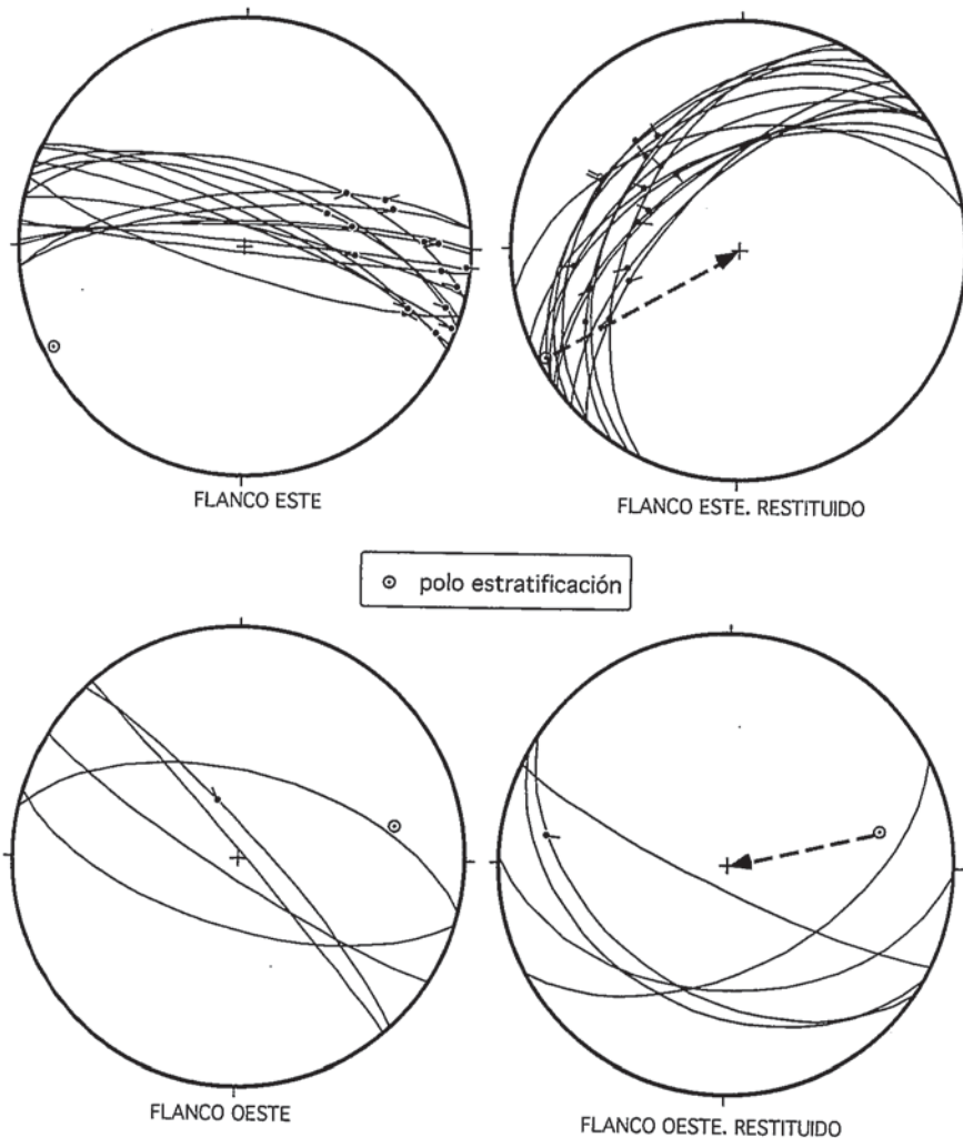
Fig. 3.- Estereogramas de las orientaciones de planos y estriás observados a escala de afloramiento sobre las fallas sinsédimentarias (izquierda) y restituidas corrigiendo el plegamiento terciario (derecha). Los círculos trazados en el mapa de la figura 1 indican las áreas de procedencia de los datos en ambos flancos del anticlinal de Campos.
