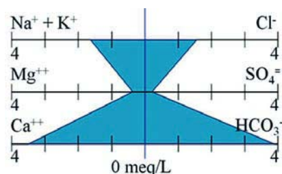
Fig. 4.- Diagrama de Stiff relativo a la composición aniónica y catiónica del agua en el sondeo Aldealegua - 2 (ALD - 2).
