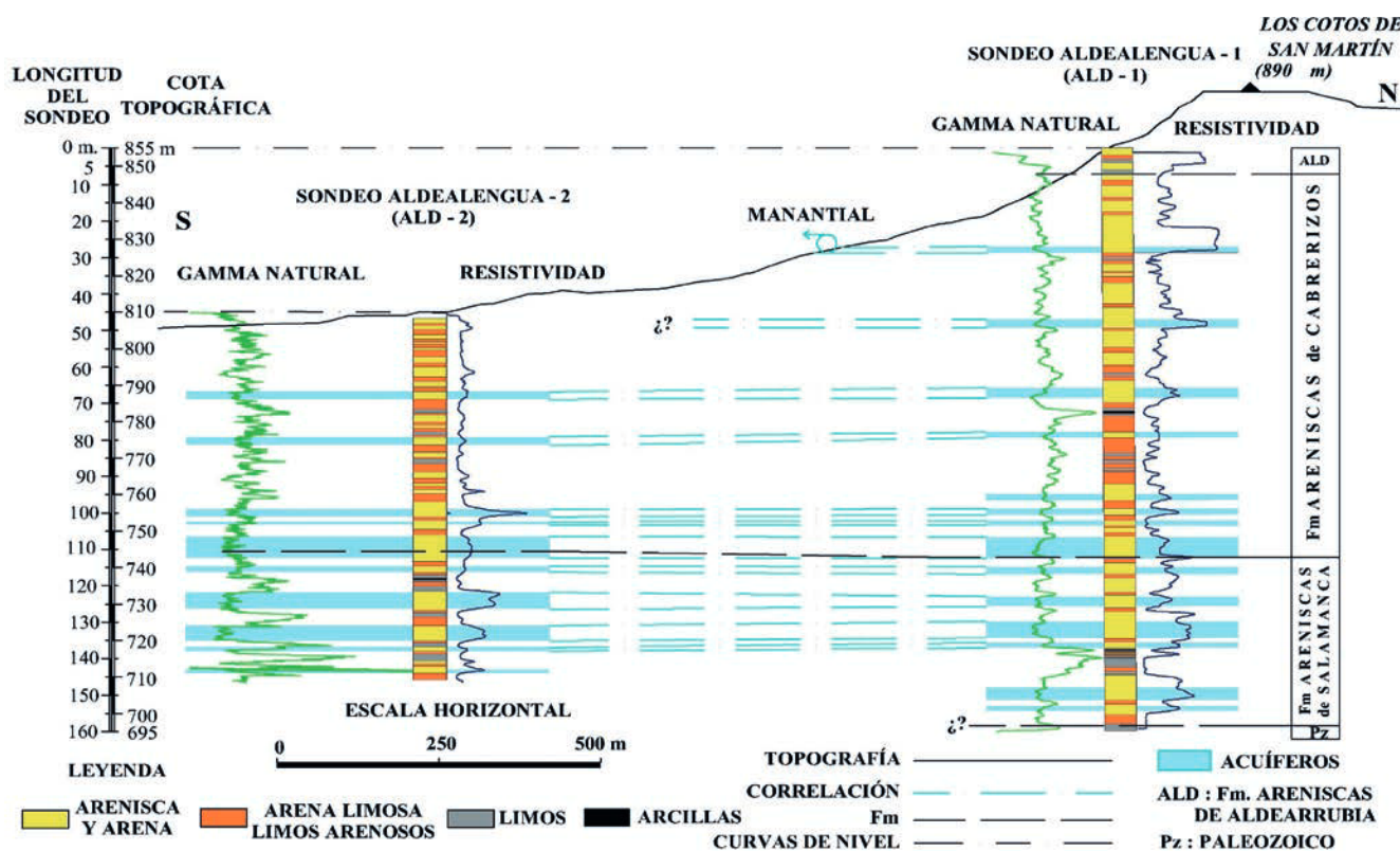
Fig. 3.- Identificación de los distintos niveles de acuíferos presentes en cada sondeo a partir de la interpretación litológica de las diagramas de resistividad y gamma natural, así como la correlación de los niveles de aguas subterráneas entre ambos pozos. Ver figura en color en la web.
