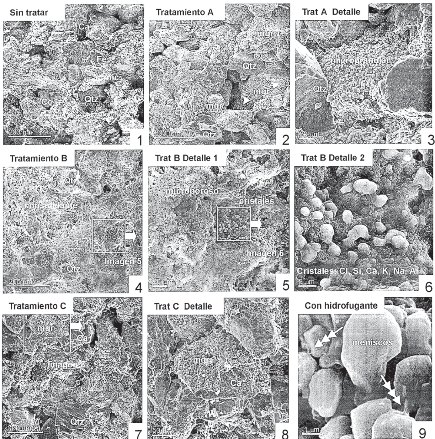
Fig. 1.- Imágenes de microscopio electrónico de barrido de la superficie de la muestra RMS-2 sin tratar y con diversos tratamientos. Cc: cemento de calcita; Ca: calcita detrítica; Qtz: clasto de cuarzo; Arc-mic: matriz arcillo micácea; Fe: óxidos de hierro; mgr: agregado microgranular.
