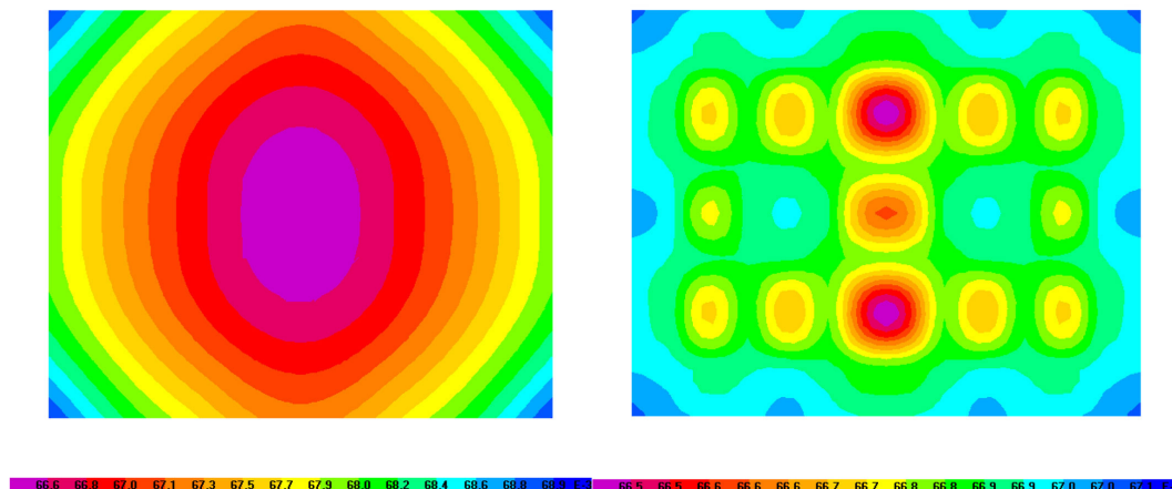
Figura 4. Gráfico de asientos. Izq.: Losa maciza 8,10 \times 6,45 (asiento máximo con acciones características 51 mm). Drcha.: Losa aligerada 8,10 \times 6,45 (asiento máximo con acciones características 49 mm).
