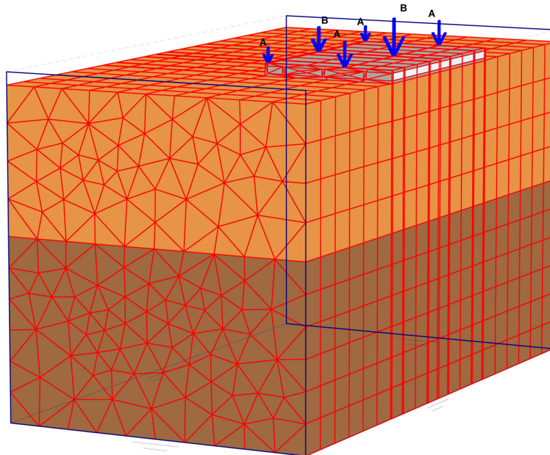
Figura 3. Modelo 3D de la losa en Plaxis 3D.
