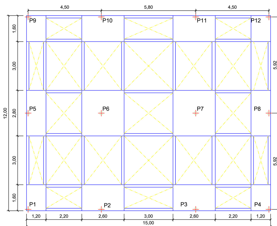
Figura 1. Esquema en planta de la cimentación estudiada. 15,00 × 12,00.
