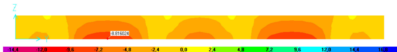
Figura 12 Componente F_{11} en nervio interior transversal de la primera línea de soportes. Losa aligerada. (Combinación Permanentes + Variables – kN/m).
