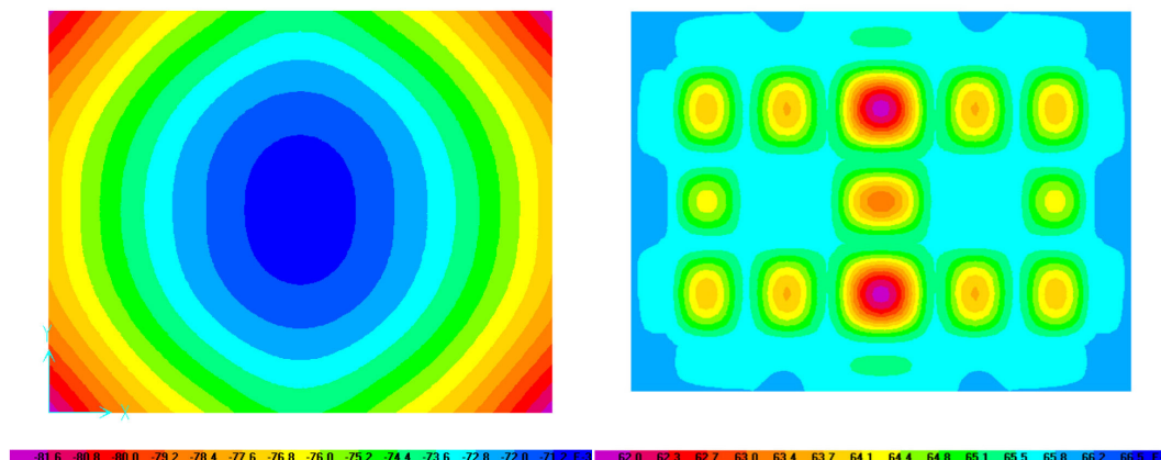
Figura 5. Gráfico de asientos. Izq.: Losa maciza 12 \times 15 (asiento máximo con acciones características 59 mm). Drcha.: Losa aligerada 12 \times 15 (asiento máximo con acciones características 48 mm).
