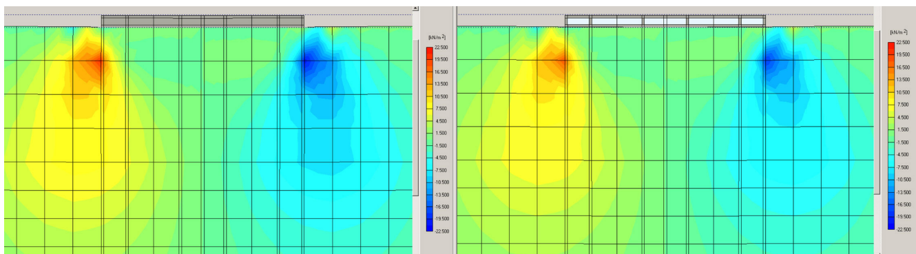
Figura 17. Resultado de tensiones de corte. Sección longitudinal por el eje de simetría.
