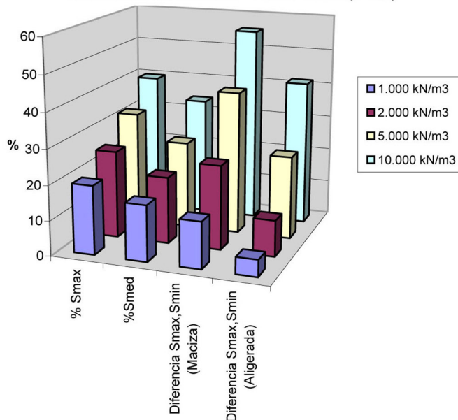
Reducción de asientos - LOSA 15x12 (Solid)
