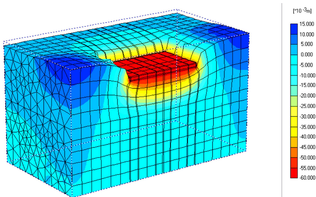
Figura 14. Deformaciones obtenidas en Plaxis para la losa maciza.
