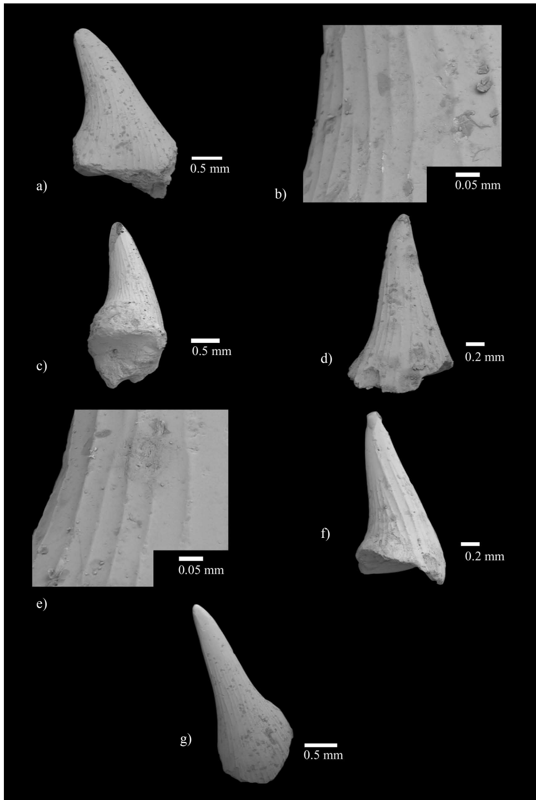
Figura 3. Dientes de Megascylorhinus miocaenicus (Antunes y Jonet, 1970) de la Formación Arenas de Huelva, España: P-C14, diente anterior en vista labial (a), detalle de estrías (b), perfil (c); P-C67-1, diente anterior vista perfil (d), detalle de estrías (e) y vista perfil (f); P-C80-1, diente anterior en vista labial (g).
