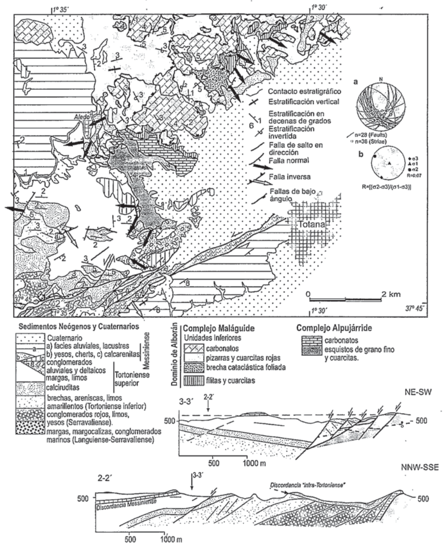
Fig. 2.- Mapa y cortes geológicos del borde oriental de la Cuenca de Lorca, área localizada en la Fig. 1. Proyecciones estereográficas, hemisferio inferior, equiangular: A) fallas normales utilizadas para determinar el tensor de esfuerzos mostrado en B). Cortes geológicos localizados en el mapa geológico.
