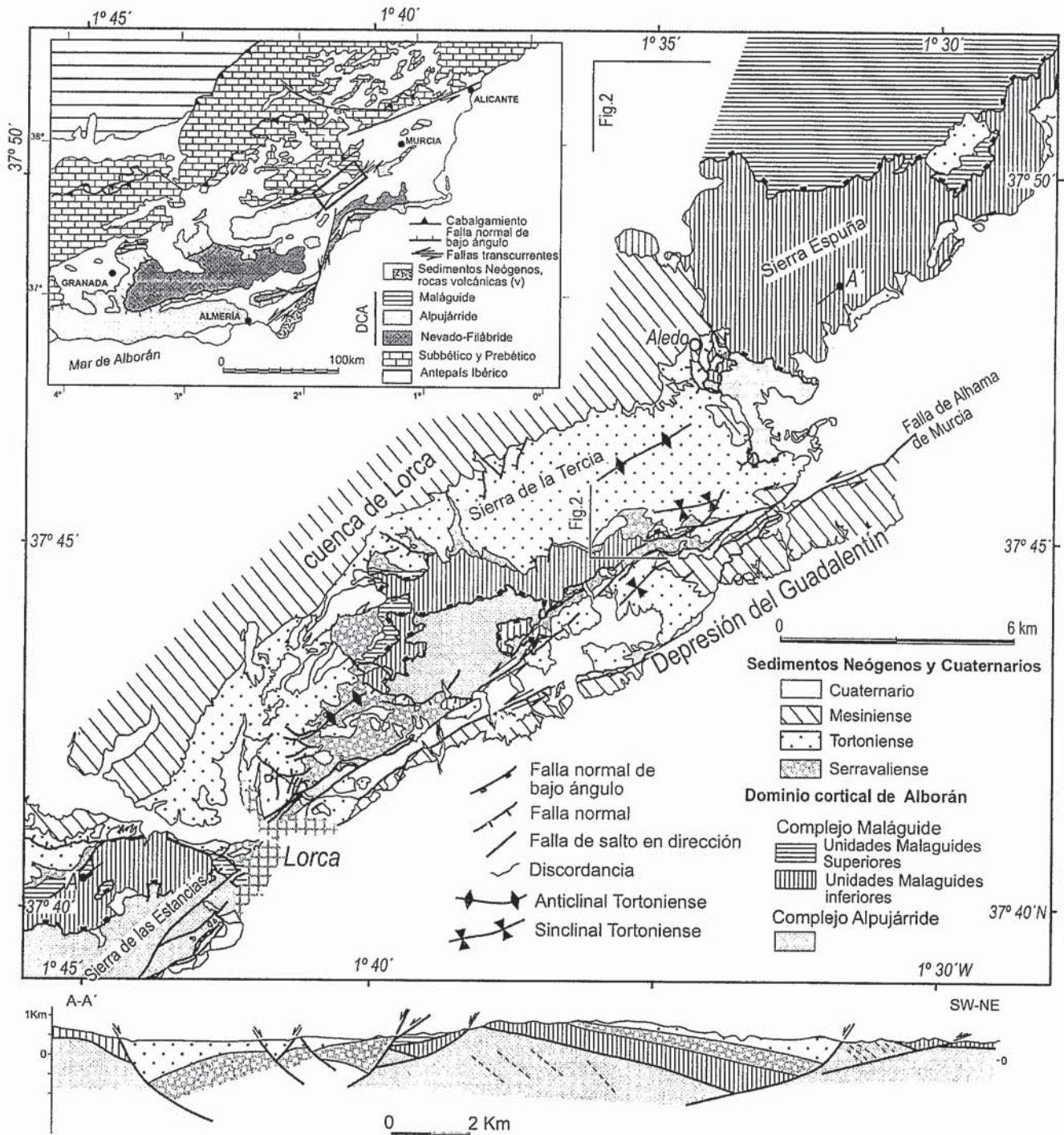
Fig. 1.- Contexto geológico de la Cuenca de Lorca, mapa geológico del área de Lorca y corte geológico del área.
