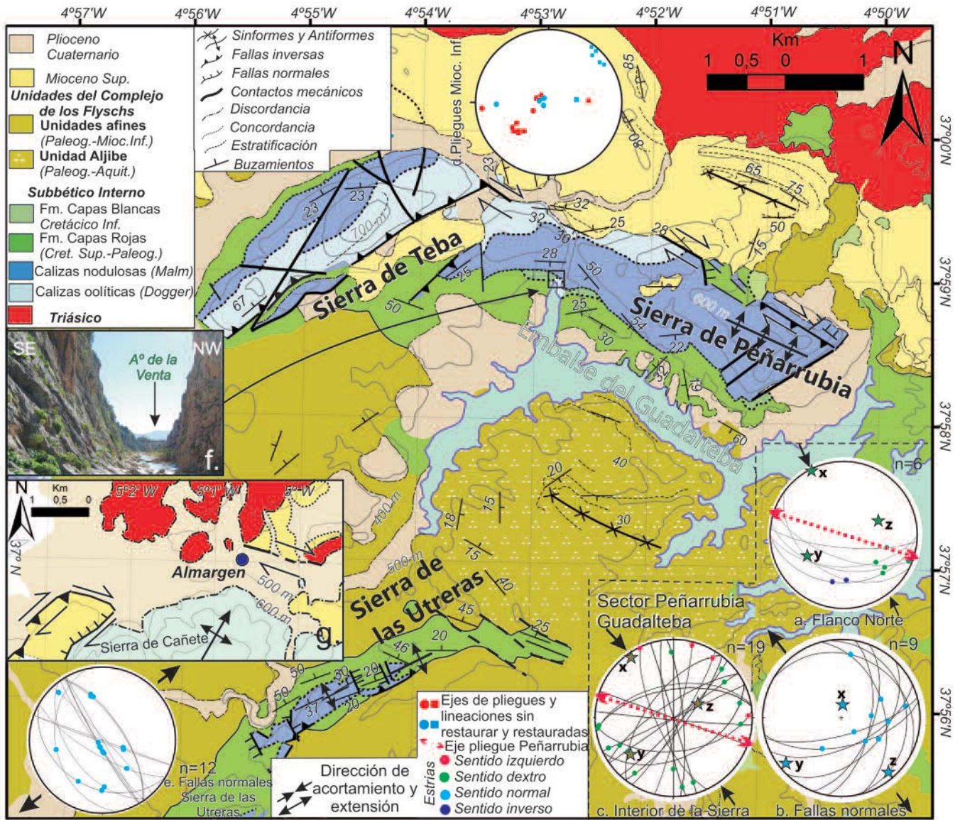
Fig. 2.- Mapa geológico del sector Teba-Peñarrubia y proyecciones estereográficas (a), (b), (c), (d) y (e). Mapa geológico del sector Almargen (g). Fig. 2.-Geological map of the Teba-Peñarrubia area and stereographic plots of the main structures (a), (b), (c), (d) and (e). Geological map of the Almargen sector (g).
