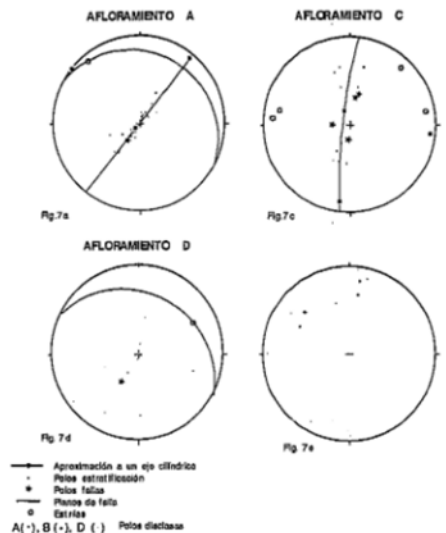
Fig 6.- Esterogramas de la estructura interna de las facies deslizadas abatidas a la horizontal. a, c, d representación de los datos de los afloramientos A, C, D. e, representación conjunta de todas las diaclasa / grietas de extensión.
