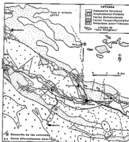
Fig 1.- Mapa geológico de la región estudiada.
