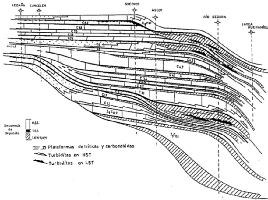
Fig. 6.- Esquema sedimentario margen-cuenca según System Tracts.
