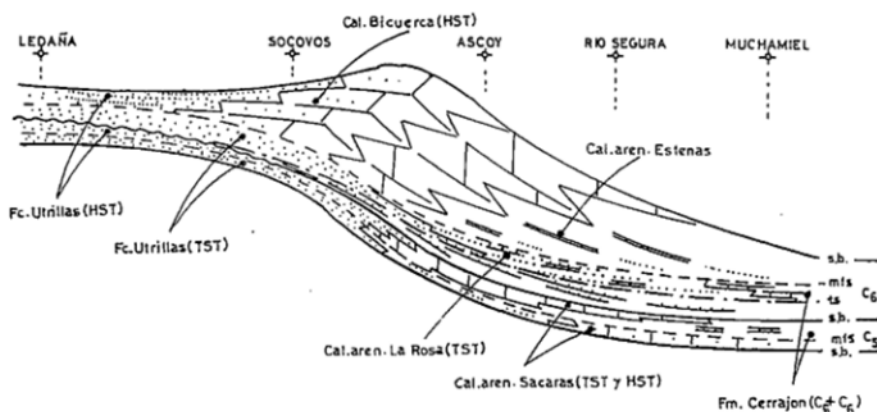
Fig. 4.- Modelo sedimentario de las Secuencias de Depósito C 5 y C 6 .
