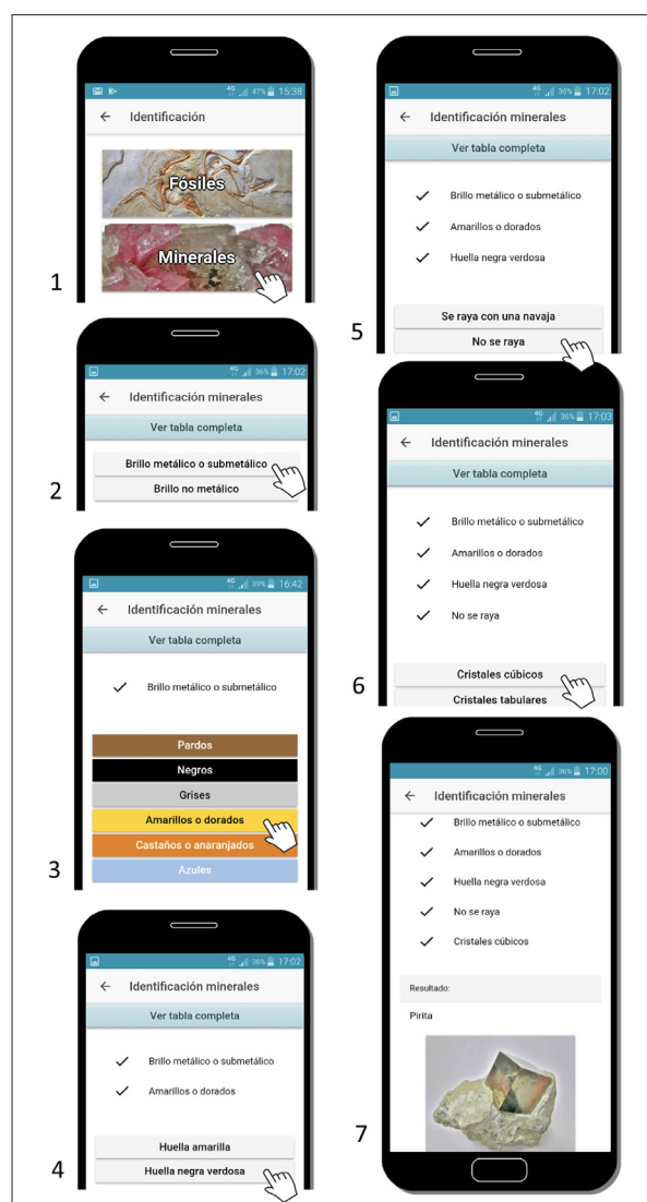
Fig. 4. (Derecha) Secuencia de pasos a seguir para identificar un mineral, en este caso la pirita.
