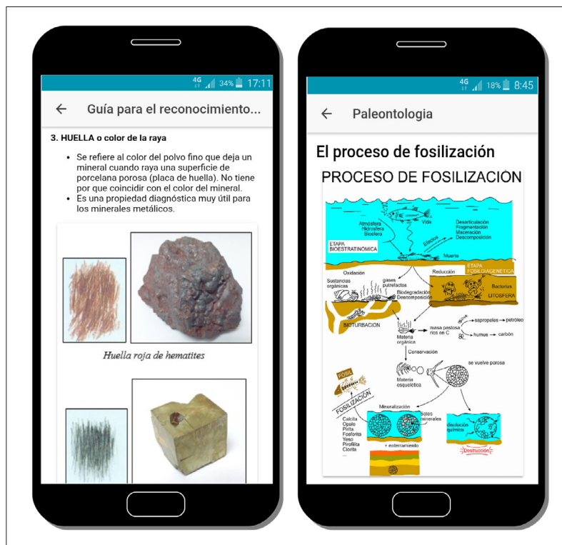
Fig. 3. (Arriba) Aspecto parcial de la guía de propiedades determinativas que se usan para el reconocimiento visual de los minerales y de un esquema didáctico ilustrativo del proceso de fosilización.
