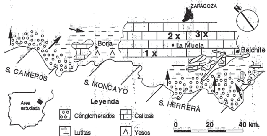
Fig. 1.- Esquema de situación y distribución de facies durante el Mioceno medio en el sector central de la Cuenca del Ebro. X: Situación de perfiles. 1: La Muela Sur, 2: La Muela Norte, 3: La Planá.
