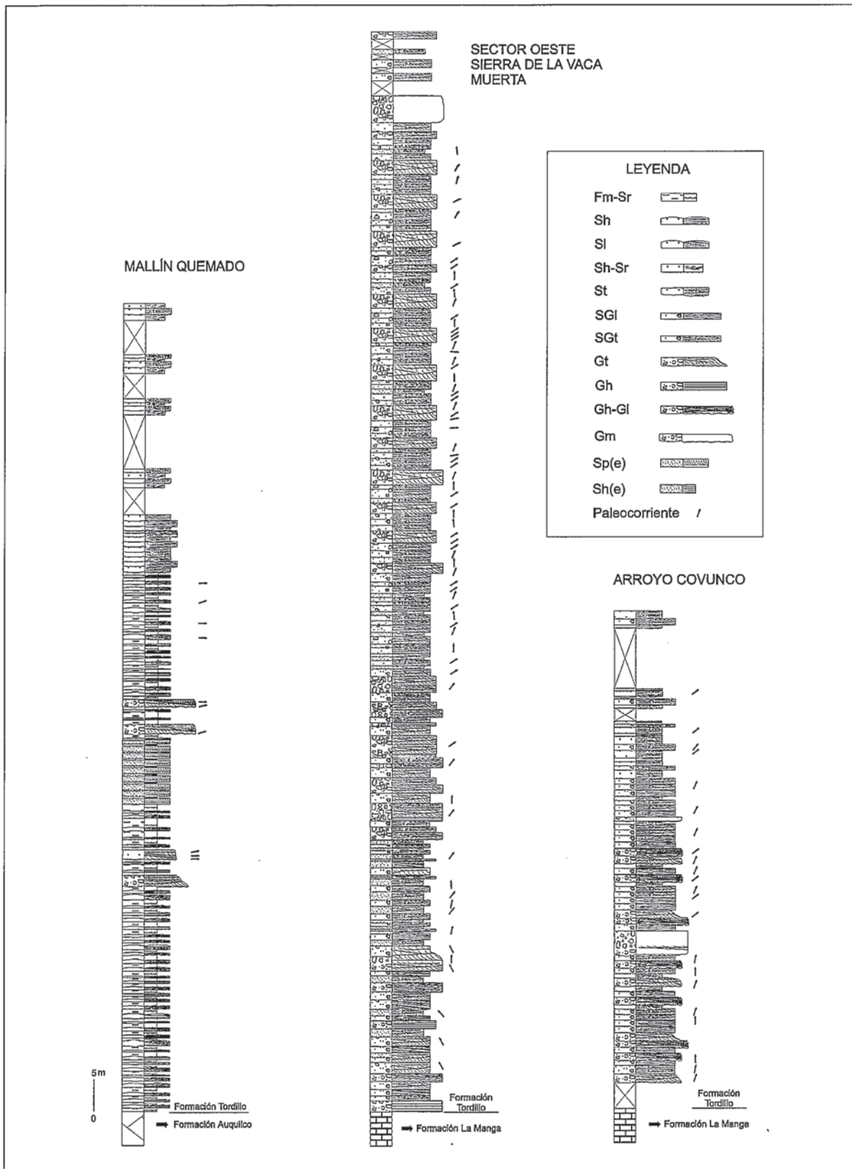
Fig. 3.- Perfiles estratigráficos de las localidades estudiadas.
