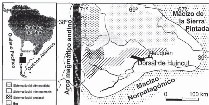
Fig. 4.- Ensayo de reconstrucción paleogeográfica para el Kimmeridgiense en el sector sur de la cuenca Neuquina (Modificado de Vergani et al, 1995).
