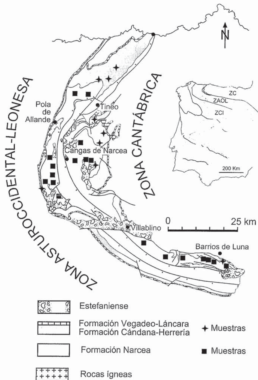
Fig. 1.- Mapa geológico simplificado con situación de las muestras: estrellas (Fm. Cándana-Herrería); cuadrados (Fm. Narcea)
