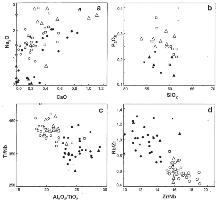
Fig. 2.- Diagramas de las pelitas cámbricas (símbolos en negro) y precámbricas (símbolos en blanco). Triángulos: ZAOL. Cuadrados: ZC. Círculos: ZCI. V. texto.
