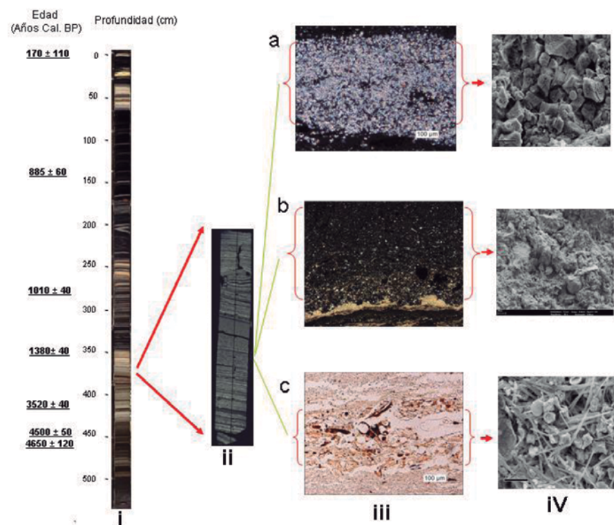
Fig. 2.- Registro sedimentario finamente laminado del lago de Montcortés; i) sondeo largo MON04-4A-1K con las dataciones ^{14}\text{C} AMS calibradas, ii) lámina delgada de una sección del sondeo, iii) imagen de microscopía óptica de las diferentes laminaciones que comprenden una varva: a) lámina de calcita, b) lámina detrítica y c) lámina orgánica, iv) imágenes de MEB de las diferentes láminas.
