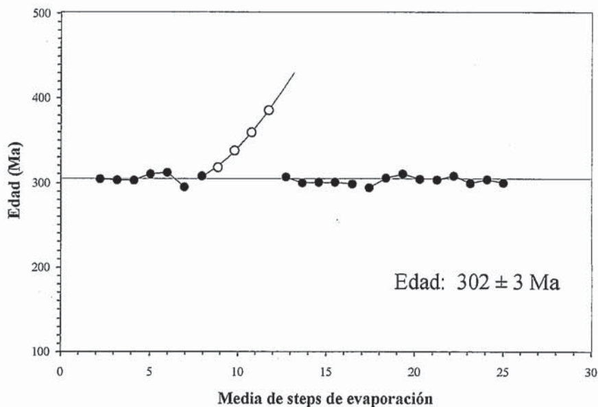
Fig. 3.- Edades ^{207}\text{Pb}/^{206}\text{Pb} en cristal único de citrón del granito de la Cabrera. Los puntos blancos indican edades mezcla del borde con un núcleo restítico.
