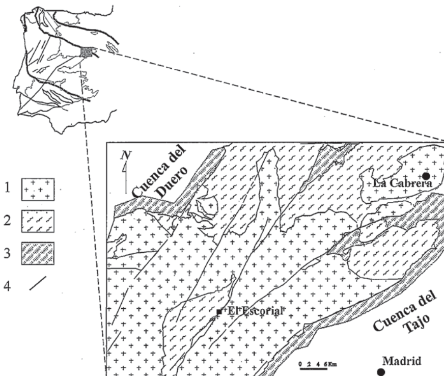
Fig. 1.- Esquema geológico de la parte oriental del Sistema Central y localización del plutón de La Cabrera: 1) Granitoides variscos, 2) Rocas metamórficas, 3) Rocas sedimentarias (cobertura mesozoica y cenozoica), y 4) Fallas.
