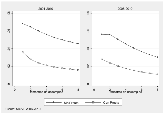
GRÁFICO 7: TASAS MEDIAS DE SALIDA DEL DESEMPELO INVOLUNTARIO CON DESPLAZAMIENTO.
