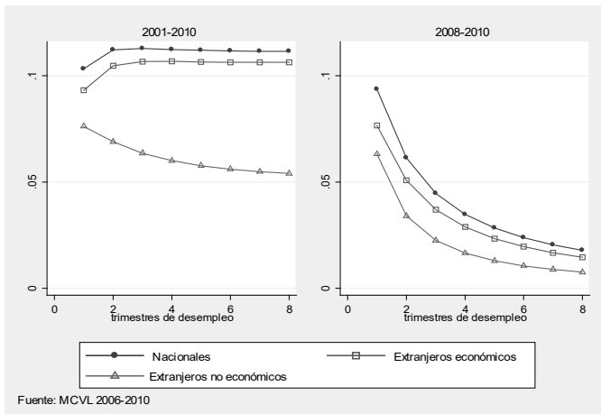
GRÁFICO 6: TASAS MEDIAS DE SALIDA DEL DESEMPEÑO VOLUNTARIO CON DESPLAZAMIENTO.
