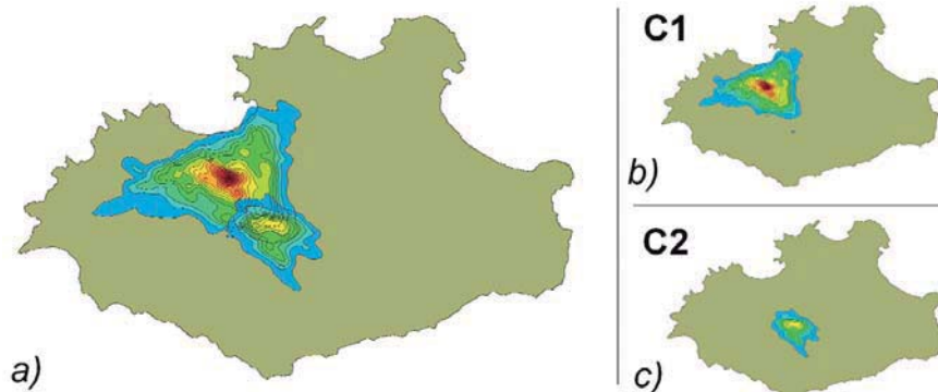
Fig. 7.- Posición de los centros de convergencia de diques C1 y C2 (b y c). Isolíneas de igual número de intersecciones de diques. Empiezan en 100 (equidistancia 100). a) Superposición de las figuras b) y c).
