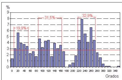
Fig. 4.- Distribución de las direcciones de los diques del Edificio São Vicente Inferior. La línea roja horizontal marca una distribución radial perfectamente homogénea.
