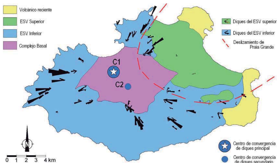
Fig. 2.- Esquema geológico de la isla de São Vicente con la distribución de los diques.
