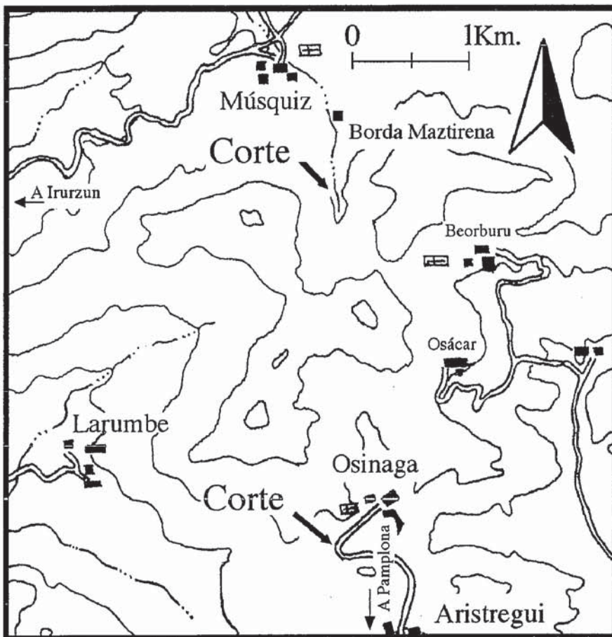
Fig. 1.- Situación geográfica de los cortes de Osinaga y Músquiz.
