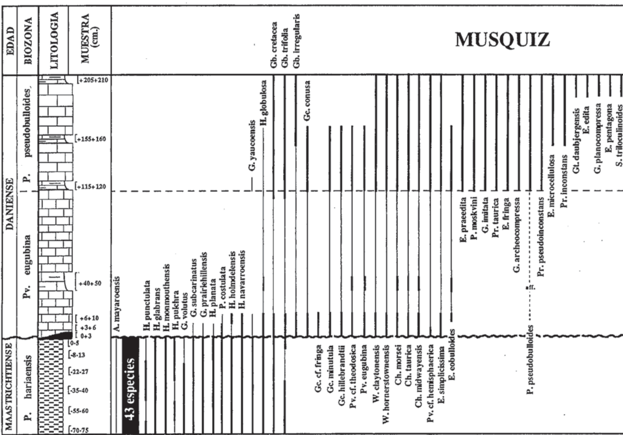
Fig. 2.- Bioestratigrafía con foraminíferos planctónicos en Osinaga y Músqiz.
