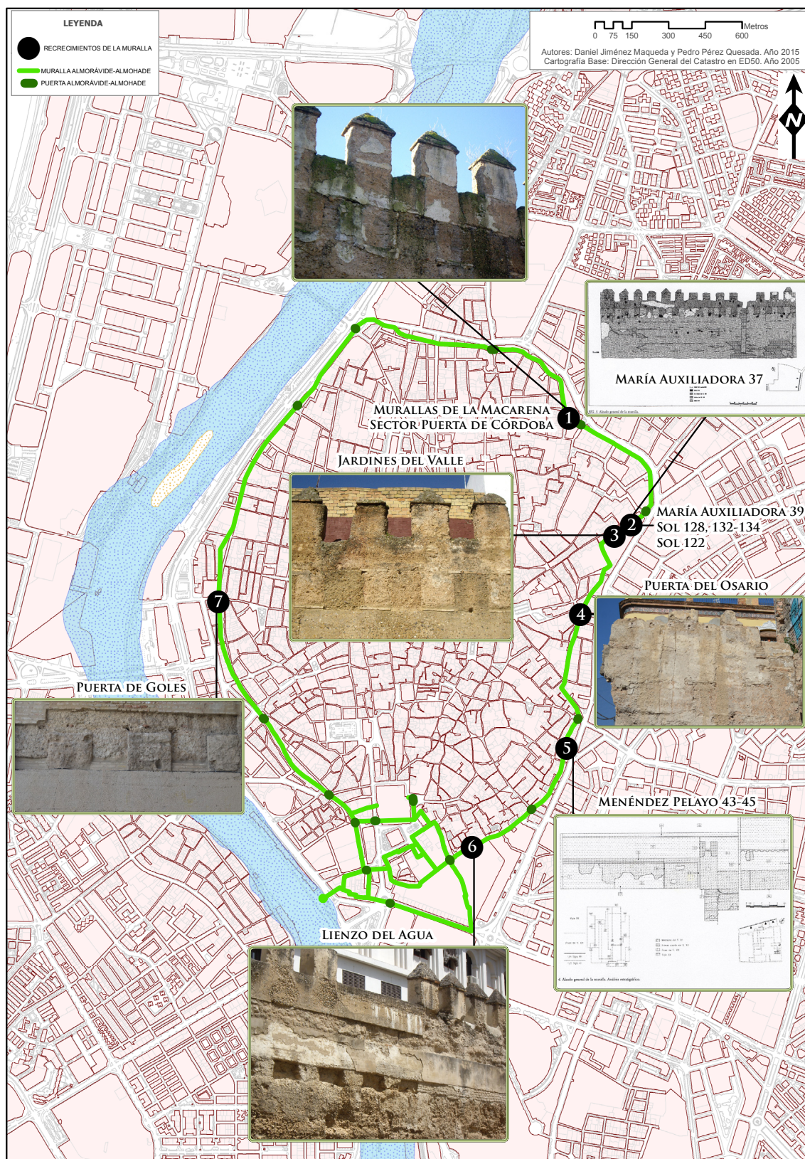
Figura 3. Puntos del recinto en los que se ha documentado el recrecimiento de la muralla.
