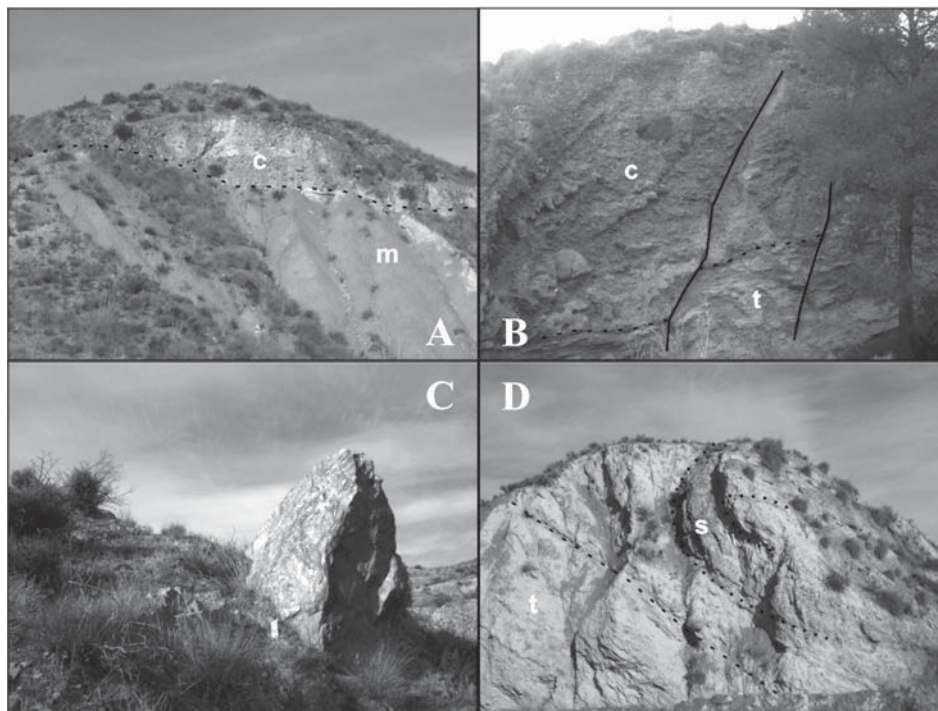
Fig. 3.- Foto A) Imagen de campo de la discordancia entre el nivel estudiado (c) y las margas bioturbadas de la base (m). Foto B) Afloramiento en el que se observan las características y espesor del nivel conglomerático (c) en discordancia sobre turbiditas (t). Foto C) Bloque de tamaño métrico perteneciente al nivel estudiado. Foto D) Foto de afloramiento de un slump (s) dentro del nivel guía sobre la secuencia turbidítica (t).
