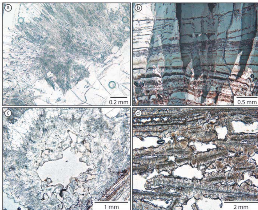
Fig. 5.- Texturas de los espeleotemas. a, c y d nicóles paralelos, b nicóles cruzados. a) Abanicos de aragonito. b) Cristales columnares de calcita con bandas de crecimiento. c) Mosaico equant de calcita cerrando la porosidad del canal central de una estalactita. d) Rafts de calcita. Ver figura en color en la web.
