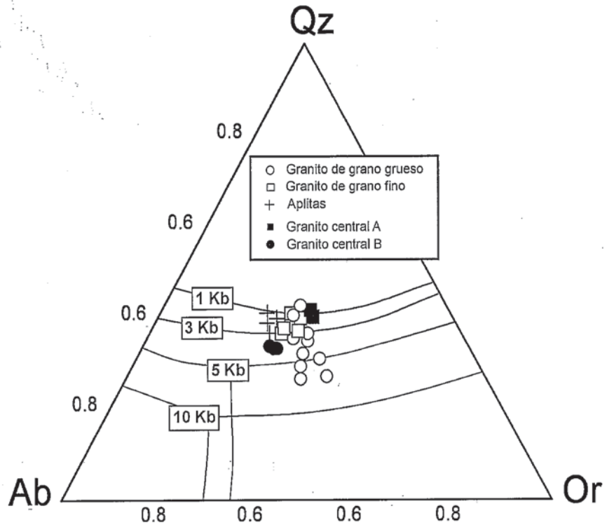
Fig. 3.- Proyección de las muestras del batolito de Nisa-Albuquerque en el diagrama triangular Qz-Ab-Or con las curvas cotécticas de Tuttle y Bowen (1958).
