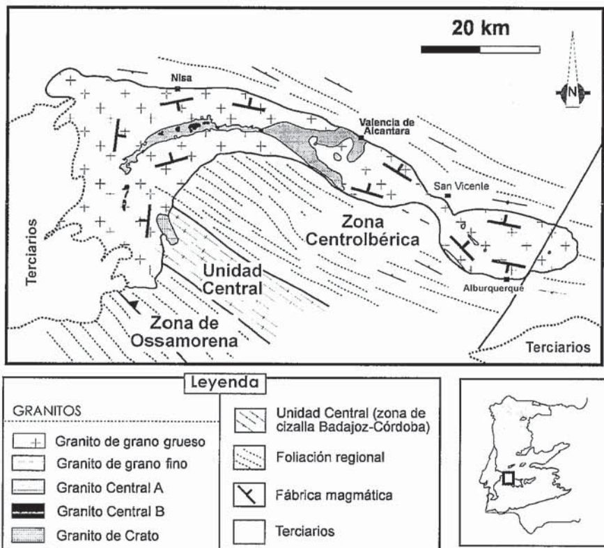
Fig. 1.- Esquema geológico del batolito de Nisa-Alburquerque (geología del encajante simplificada)
