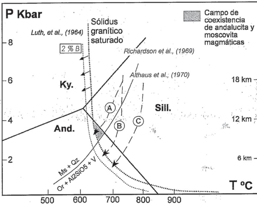
Fig. 2.- Esquema P-T con tres posibles trayectorias de ascenso y emplazamiento. Curvas de estabilidad de aluminosilicatos de Richardson et al., (1969). Curva de estabilidad de la moscovita de Althaus et al., (1970). Sólidos granítico saturado de Luth, (1964).
