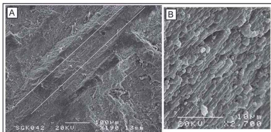
Fig. 4.- A) Microestructura en conchas de Chondrodonta sp.: A) Corte transversal. Las líneas blancas representan las líneas de crecimiento. B) Detalle de las escamas que componen la microestructura.
