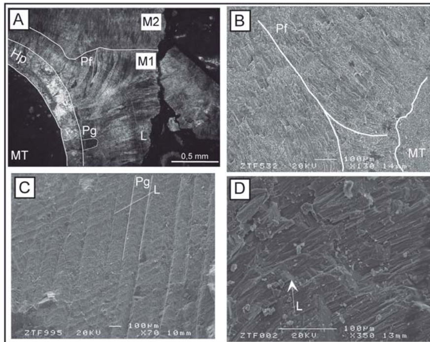
Fig. 2.- Microestructuras en conchas de rudistas monopléuridos: A) Corte transversal de la concha en lámina delgada (XPL, nículos cruzados) donde se observa la matriz micrítica (MT), el hipostracum de la concha (Hp) y el miostracum de dos individuos (M1 y M2). En M1 aparecen resaltados los prismas gruesos (Pg) y los prismas finos (Pf), al igual que las líneas de crecimiento (L). B) Imagen de SEM de los prismas finos (Pf) del miostracum en corte longitudinal, que se abren en abanico hacia la matriz micrítica (MT) C) Detalle al SEM de los prismas gruesos (Pg) del miostracum, en corte oblicuo, con las líneas de crecimiento (L). D) Detalle al SEM de los prismas finos del miostracum con las líneas de crecimiento (L).
