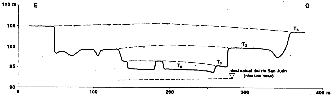
Fig. 3.- Disposición geométrica de las terrazas en un corte transversal al río Albarraçín (Línea A-B en la fig. 2). Obsérvese el carácter convexo de la superficie de las terrazas.
