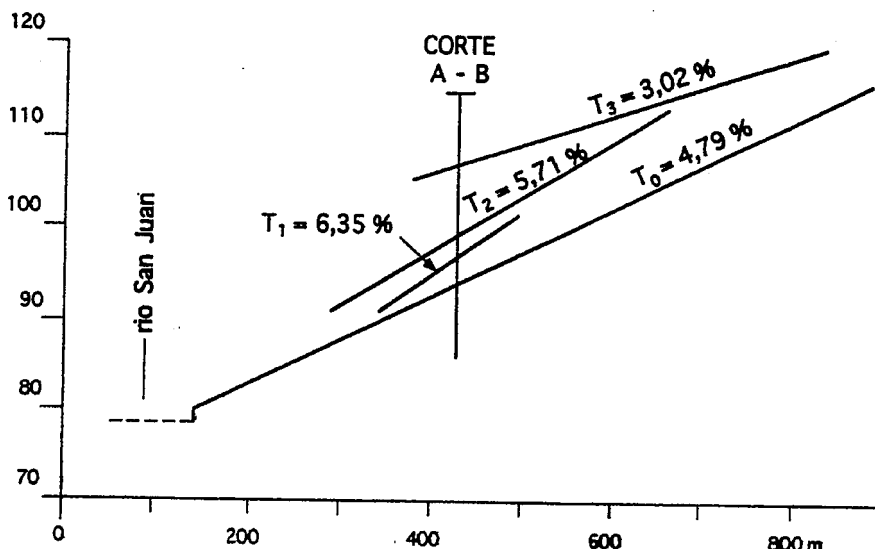
Fig. 4.- Perfiles longitudinales de las superficies de las terrazas del margen derecho del río Albarracín en la zona de confluencia con el río San Juan. Obsérvese el incremento gradual de las pendientes a medida que las terrazas son mas modernas. La terraza T0 muestra una inclinación menor, lo que sugiere que no se halla todavía en equilibrio. Valores de las pendientes expresados en %.
