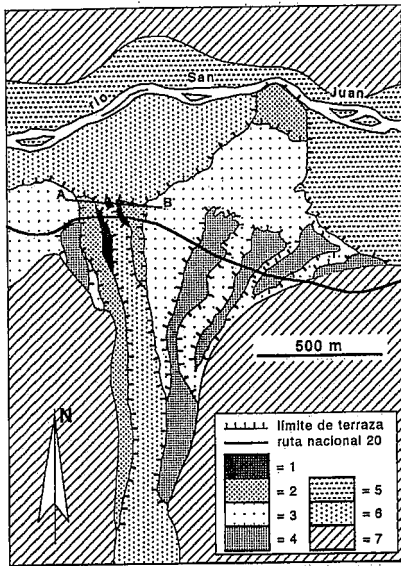
Fig. 2.- Mapa de disposición de las terrazas en la confluencia de los ríos Albarraçín y San Juan. El área cartografiada corresponde a la zona recuadrada de la fig. 1B. 1 = terraza T1. 2 = terraza T2. 3= terraza T3. 4= terraza T4. 5 = terraza actual del río San Juan. 6 = terraza actual del río Albarraçín (T0) y 7 = substrato. La línea A-B indica la localización del corte transversal representado en la fig. 3.
