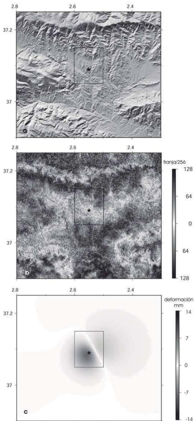
Fig. 4.- A) Modelo digital del terreno de la zona de estudio B) Interferograma cosísmico realizado a partir de una imagen tomada antes del terremoto (05/10/1999) y una imagen posterior (20/08/2002). C) Modelo de deformación para el terremoto de Gergal. Símbolos: estrella negra: epicentro del terremoto de Gergal; recuadro negro: zona del epicentro.
