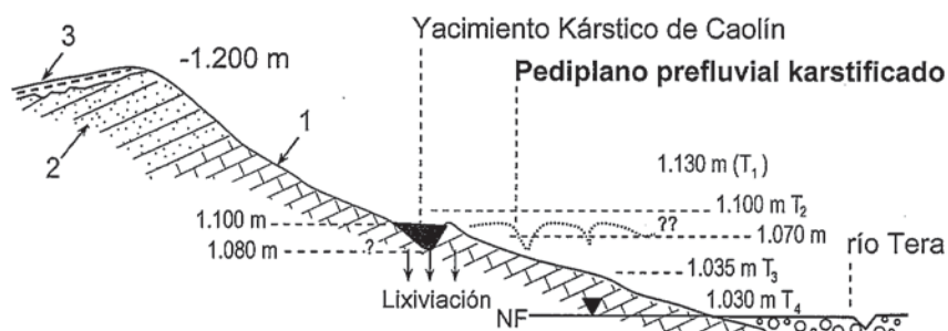
Fig. 3.- Localización geomorfológica del yacimiento kárstico de caolín de Chavaler (Soria) 1. Facies Purbeck-Weald: Grupo Oncala (calizas). 2. Grupo Urbión (areniscas). 3. Coluvios. T_1 , T_2 , T_3 , T_4 . Terrazas del río Tera.
