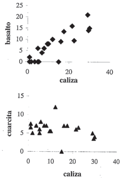
Fig. 4.- Diagramas de correlaci3n entre las dimensiones de los clastos de caliza con los de basalto y cuarcita, para cada cuerpo de A4 sup. (perfil Calçada de Carriche).
