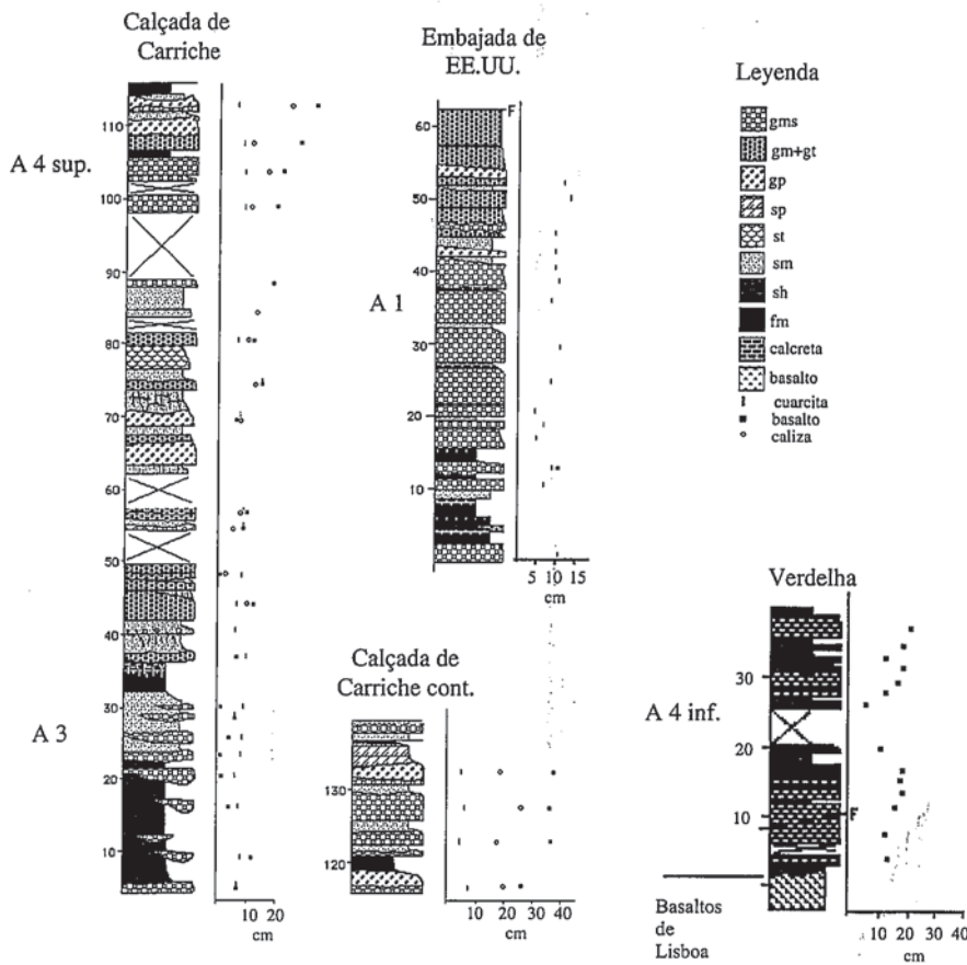
Figura 3.- Perfiles principales del Complejo de Benfca. Est representada la evoluci3n del centil, para distintos clastos.
