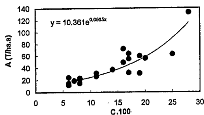
Fig. 3.- Relación pérdidas de suelo - factor de cubierta vegetal (C.100), según la U.S.L.E., para las 20 subcuencas consideradas en la cuenca del Guadalfeo vertientes al embalse de Rules
