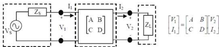
Figura 1. Matriz de transmisión de una red de dos puertos. Fuente: Adaptado de (Masood & Baig, 2016).
