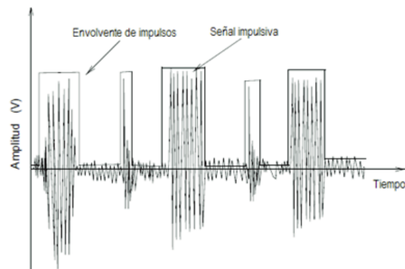
Figura 5. Envoltura de impulsos y señal impulsiva. Fuente: Adaptado de (Hrasnica, Hadine & Lehnert, 2004).
