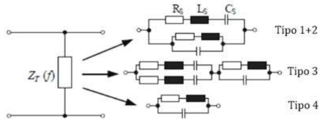
Figura 2. Modelado de impedancias con circuitos resonantes. Fuente: Adaptado de (Masood & Baig, 2016).
