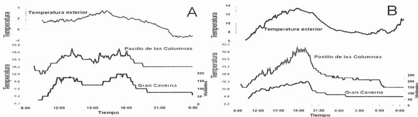
Fig. 2.- Variación temporal de la temperatura en el exterior e interior de la cavidad y distribución de los visitantes el día 22 (A) y el 29 de Abril (B).
