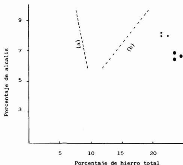
Fig. 9.—Relación entre el contenido en álcalis y hierro total de las series illita-esmectita (a) y glauconita-esmectita (b) (Velde y Odin, 1975). ● Muestras de Aznalcollar. * Muestras de Bonares.
