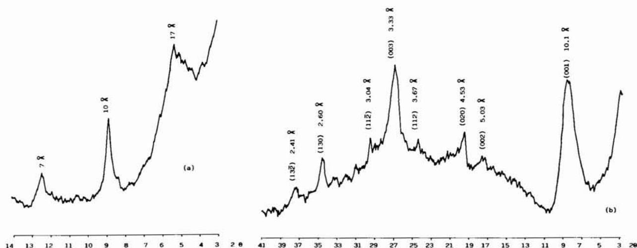
Fig. 7.—Difractogramas tipo de agregado orientado con etilenglicol de la fracción menor de 20 \mu (a) y de polvo para la mica glauconítica purificada (b). Sección de Bonares.
