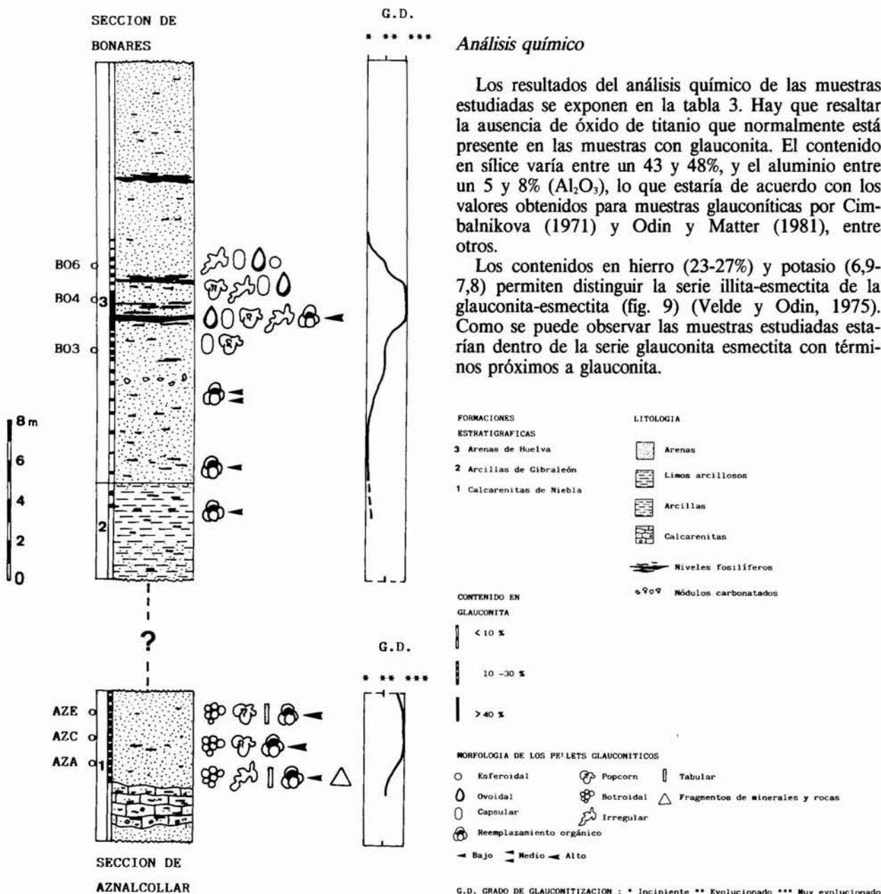
Fig. 2.—Perfiles tipo de las secciones de Bonares y Aznalcollar.
