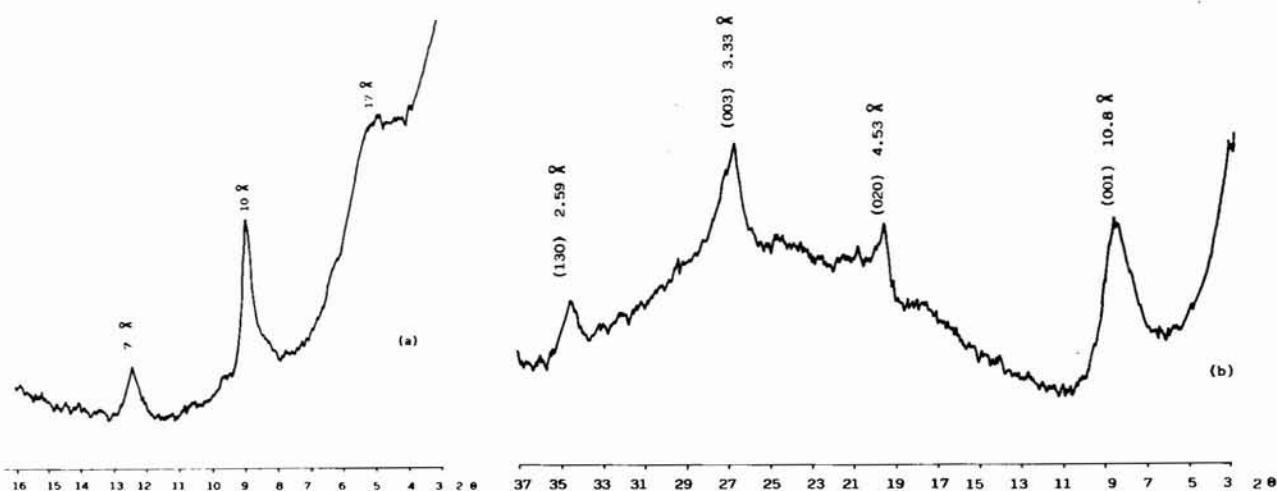
Fig. 8.—Difractogramas tipo de agregado orientado con etilenglicol de la fracción menor de 20 \mu (a) y de polvo para la mica glauconítica purificada (b). Sección de Aznalcollar.
