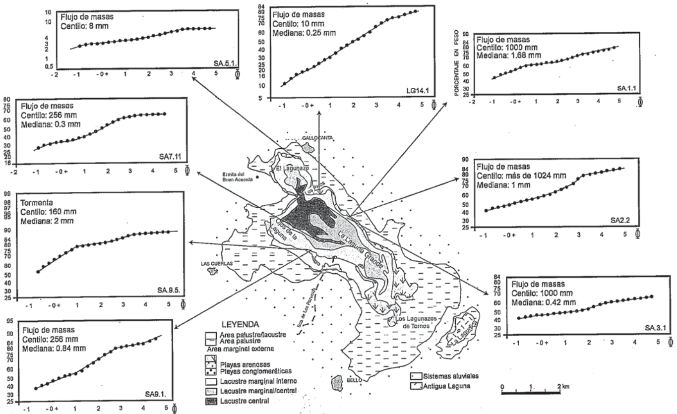
Fig. 2.- Distribuciones granulométricas correspondientes a muestras tomadas a partir de sondeos. En cada una de ellas podemos ver el centilo y la mediana obtenido para cada curva así como el proceso sedimentario interpretado.
