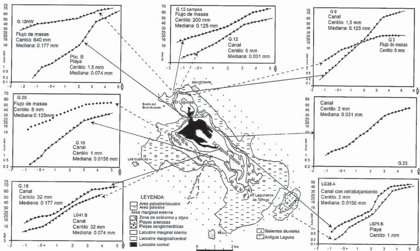
Fig. 3.- Distribuciones granulométricas correspondientes a muestras superficiales en diferentes sectores de la laguna. En cada una de ellas podemos ver el centilo y la mediana obtenido para cada curva así como el proceso sedimentario interpretado.
